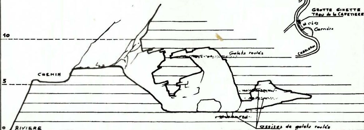
COUPE de la GROTTE GINETTE
