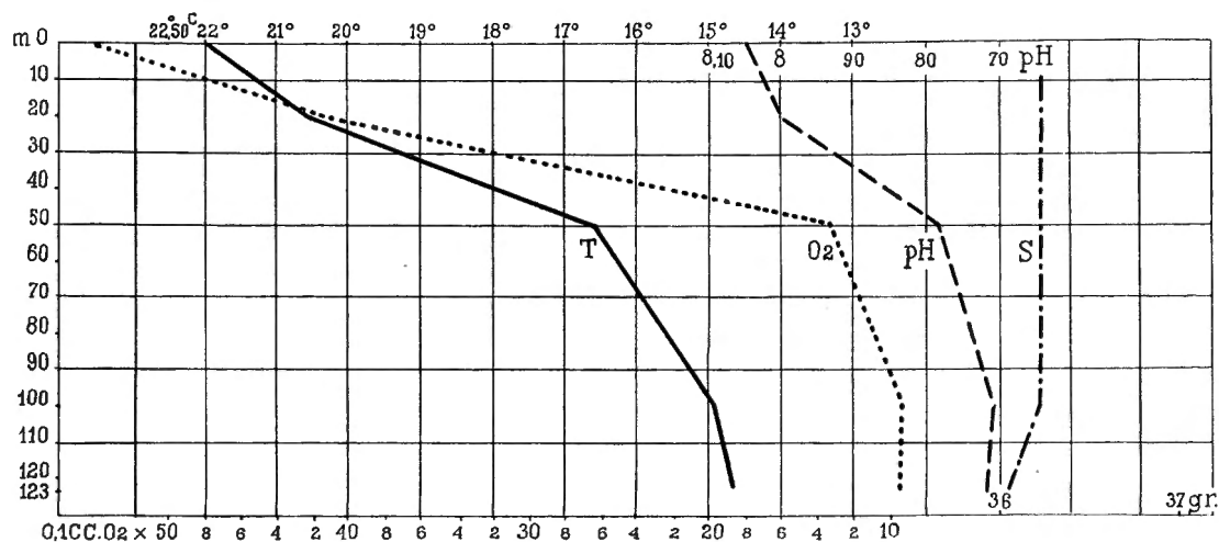
FIG. 38. — Graphique de la st. 72 bis . Variations de la température, de l'oxygène, du pH et de la salinité en fonction de la profondeur.
