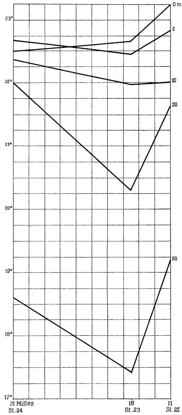
FIG. 12. — Variation de la température à 0, 5, 10, 20 et 50 m en fonction de la longitude.
