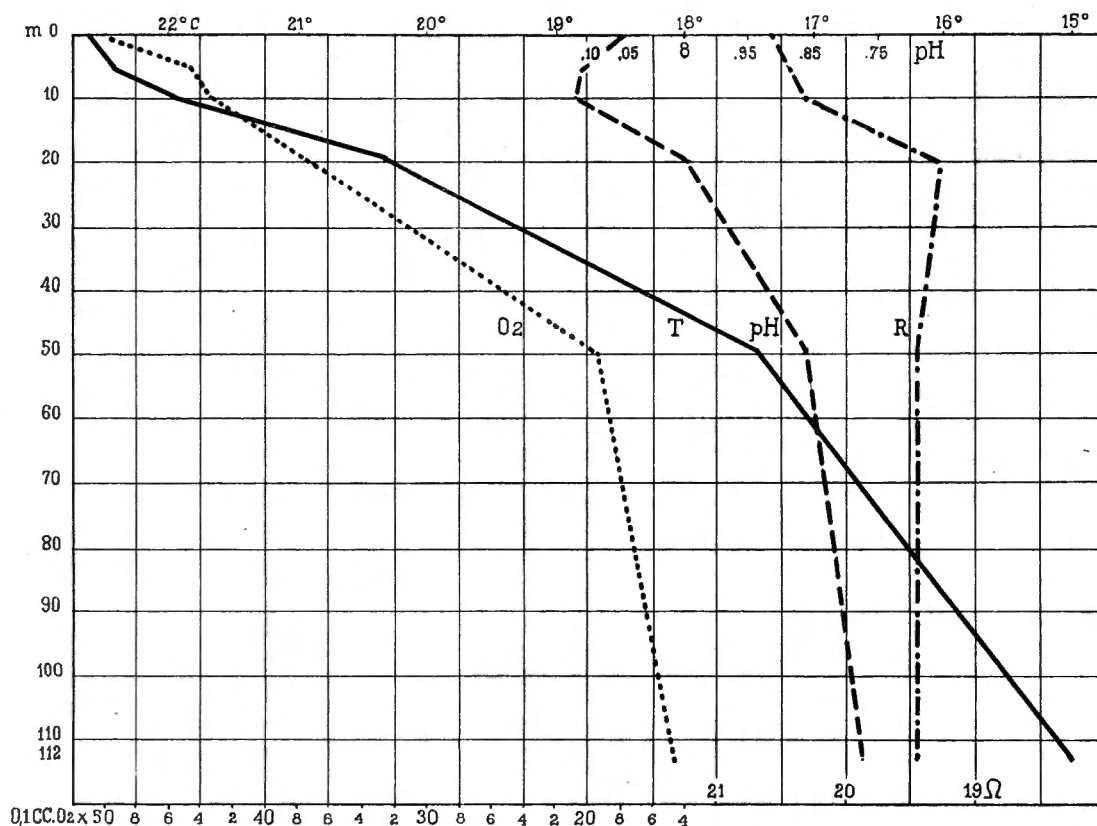
FIG. 11. — Graphique de la st. 23.
