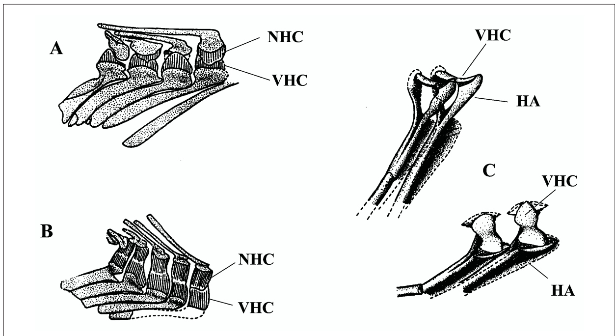
Figure 4. Chordacentra : vhc : hemichordacentra ventral; nhc : hemichordacentra neural; ha : arches hémales. a) Pholidophorus bechei , d'après Patterson, 1968. b) Pholidolepis dorsetensis , d'après Patterson, 1968. c) Tetragonolepis semicineta , d'après Thies, 1991.
