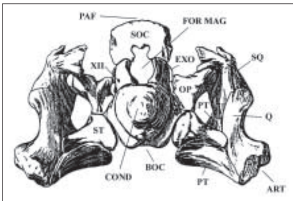
Figure 5. : Reconstruction de la région postérieure du crâne d' Ophthalmosaurus , vue de l'arrière.
