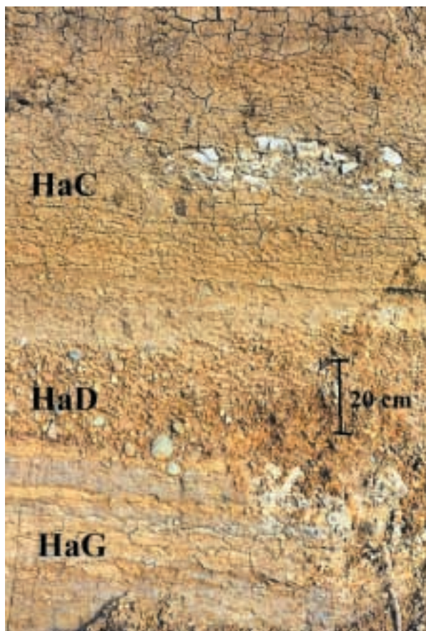
Figure 3. Coupe des Coeuvs : niveaux de haut en bas : HaC : marnes avec niveau de rognons calcaires ; HaD : niveau de galets ; HaG : marne sableuse feuilletée.
