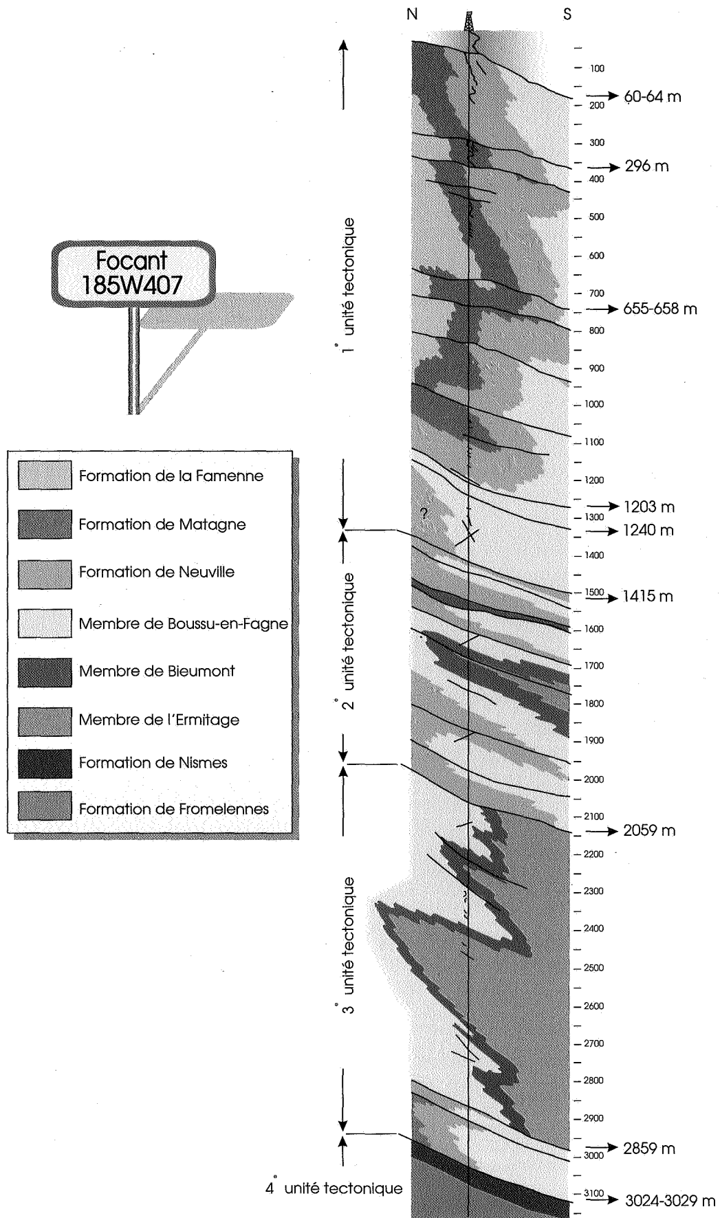
Figure 8. Coupe synthétique globale du sondage 185W407 de Focant.
