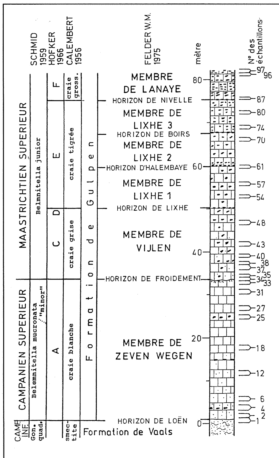
Text-Fig. 3: Lithologie, biostratigraphie et échantillonnage d'Halembaye.
