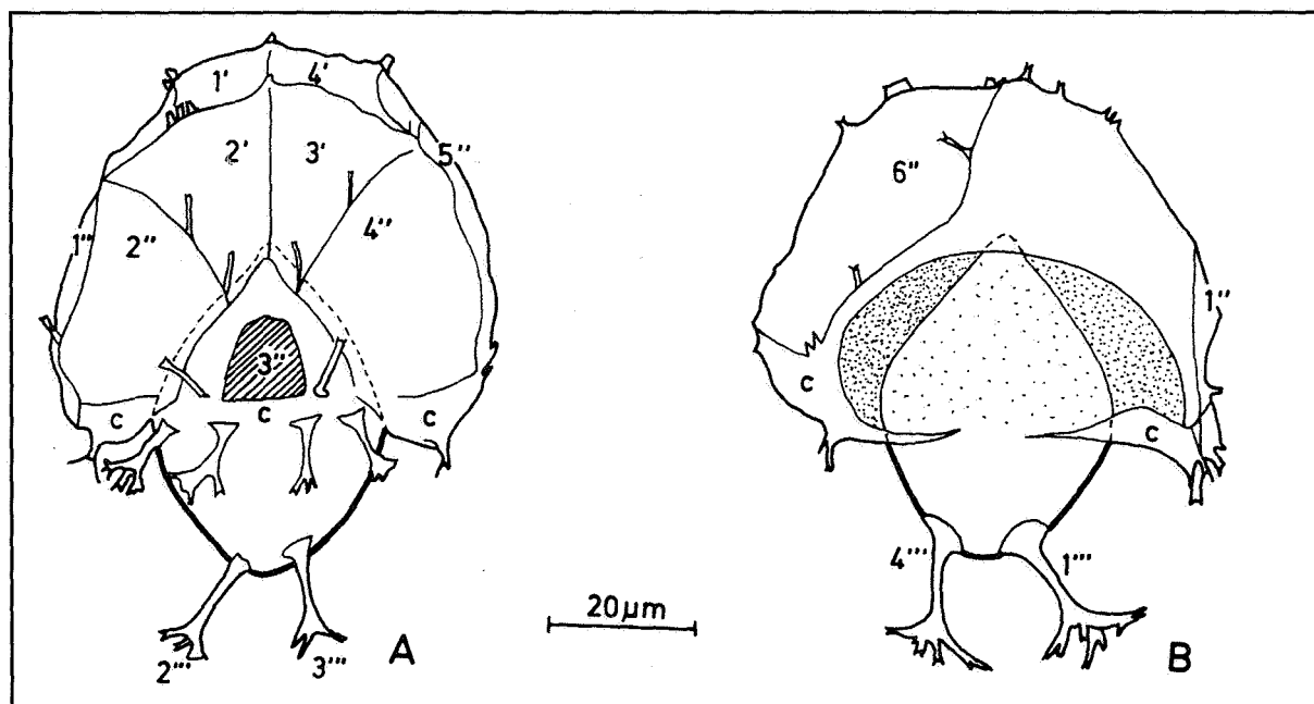
Text-Fig. 6: Flandrecysta furcata sp. nov., holotype. A, face dorsale en vue externe; B, face ventrale en vue externe.
