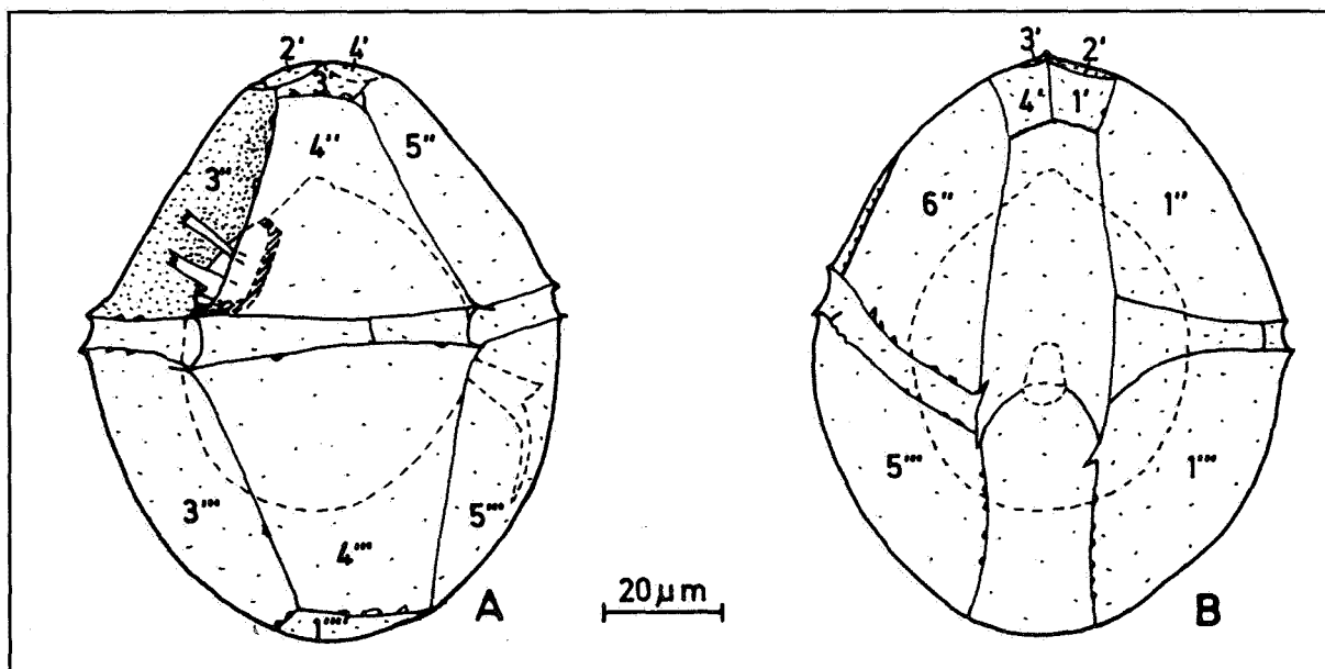
Text-fig. 11: Représentation schématique de Wilsonisphaera petila (CORRADINI 1973) comb. nov.; A, face latérale droite en vue externe; B, face ventrale en vue externe.
