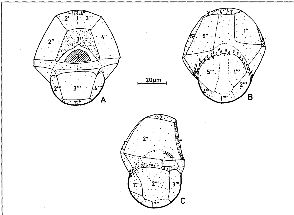
Text-fig. 8: Turnhosphaera hypoflata (YUN 1981) comb. nov.; A, face dorsale en vue externe; B, face ventrale en vue externe; C, face latérale gauche en vue externe.
