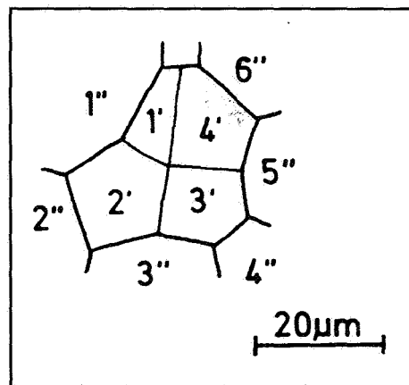
Text-fig. 10: Représentation schématique de la paratabulation de la face apicale en vue externe du genre Turnhosphaera g. nov.
