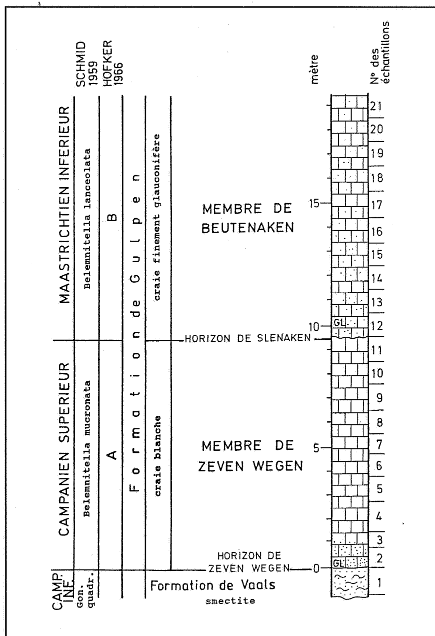
Text-Fig. 2: Lithologie, biostratigraphie et échantillonnage dans la carrière de Beutenaken (GL = glauconie).
