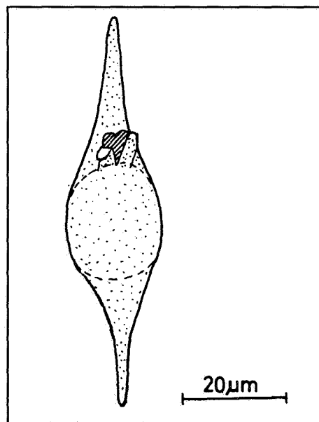
Text-fig. 14: Représentation schématique d' Ithnacysta elongata sp. nov., face dorsale en vue externe.
