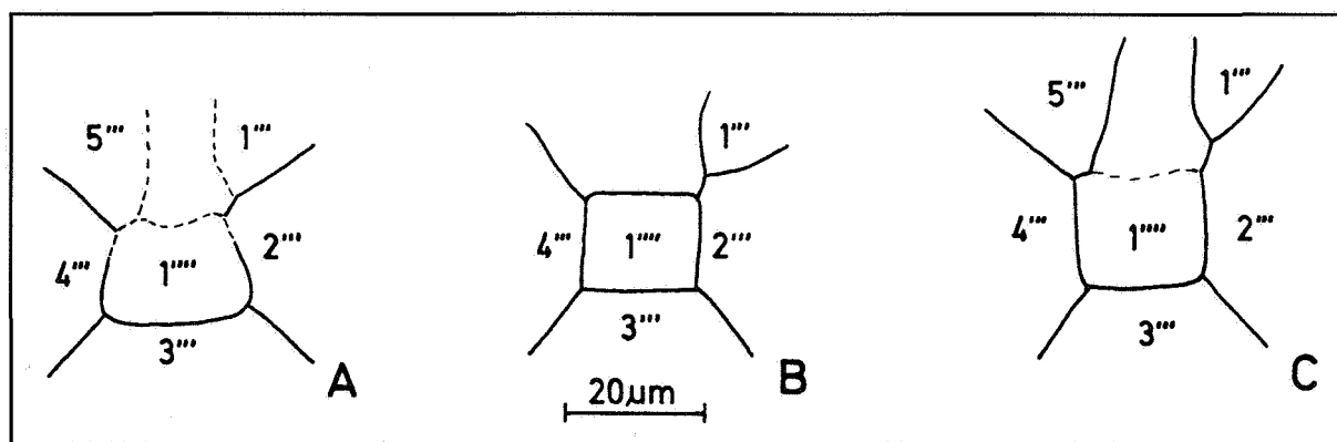
Text-fig. 9: Représentation schématique de la paratabulation de la face antapicale en vue externe; A, Turnhosphaera hypoflata (YUN 1981) comb. nov.; B, Turnhosphaera hyalina sp. nov.; C, Turnhosphaera granulata sp. nov.
