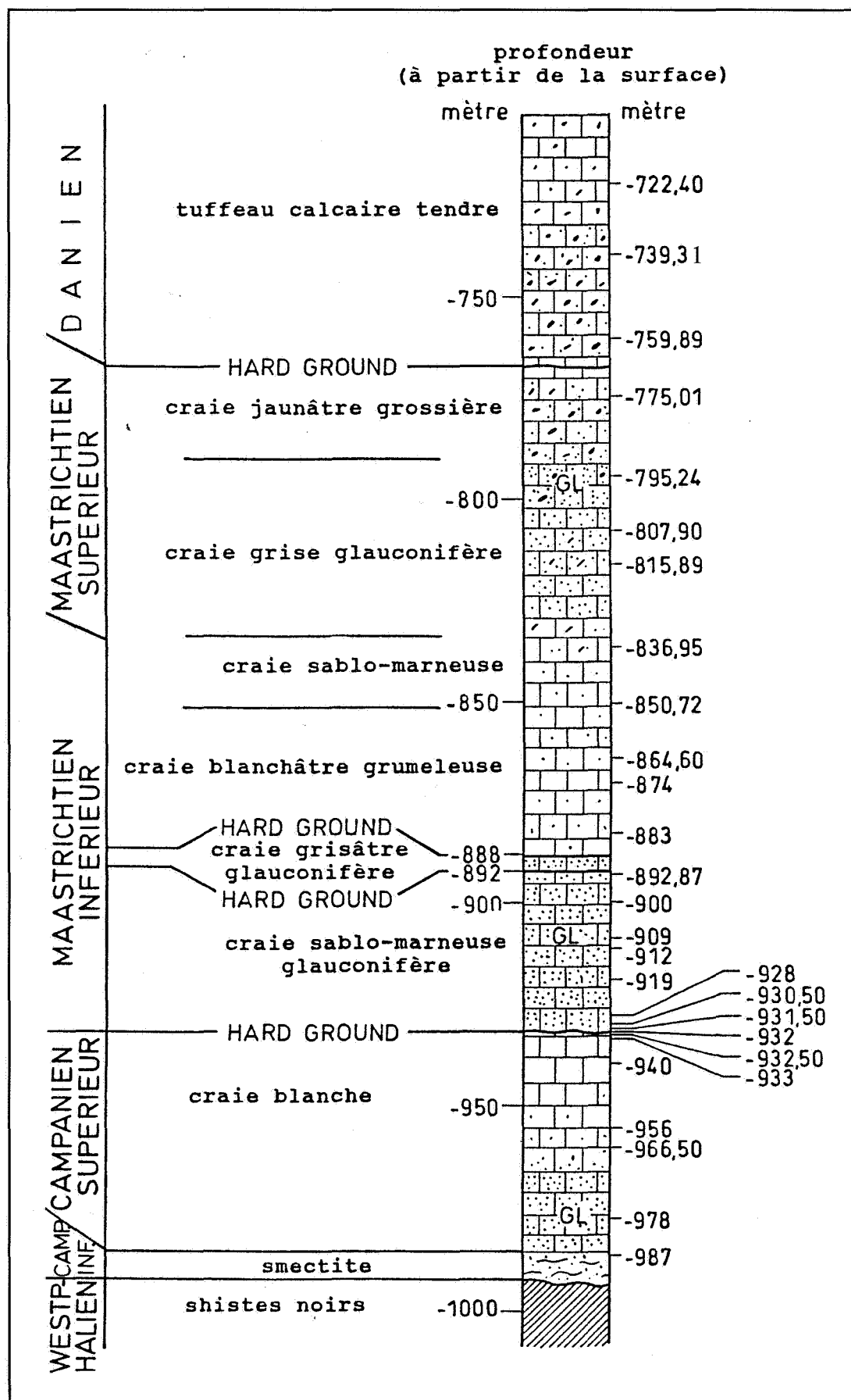
Text-fig. 4: Lithologie et échantillonnage dans le sondage de Turnhout (GL = glauconie).
