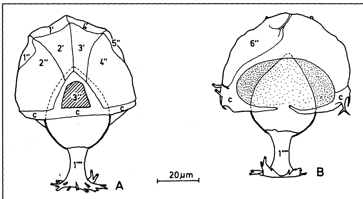
Text-fig. 7: Flandrecysta tubulosa sp. nov., holotype. A, face dorsale en vue externe; B, face ventrale en vue externe.
