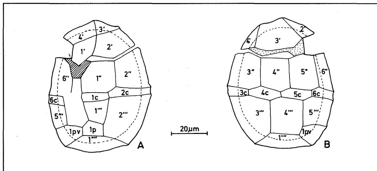
Text-fig. 5: Représentation schématique de Membranigonyaulax wilsonii sp. nov., holotype; A, face ventrale gauche en vue externe; B, face dorsale droite en vue externe.
