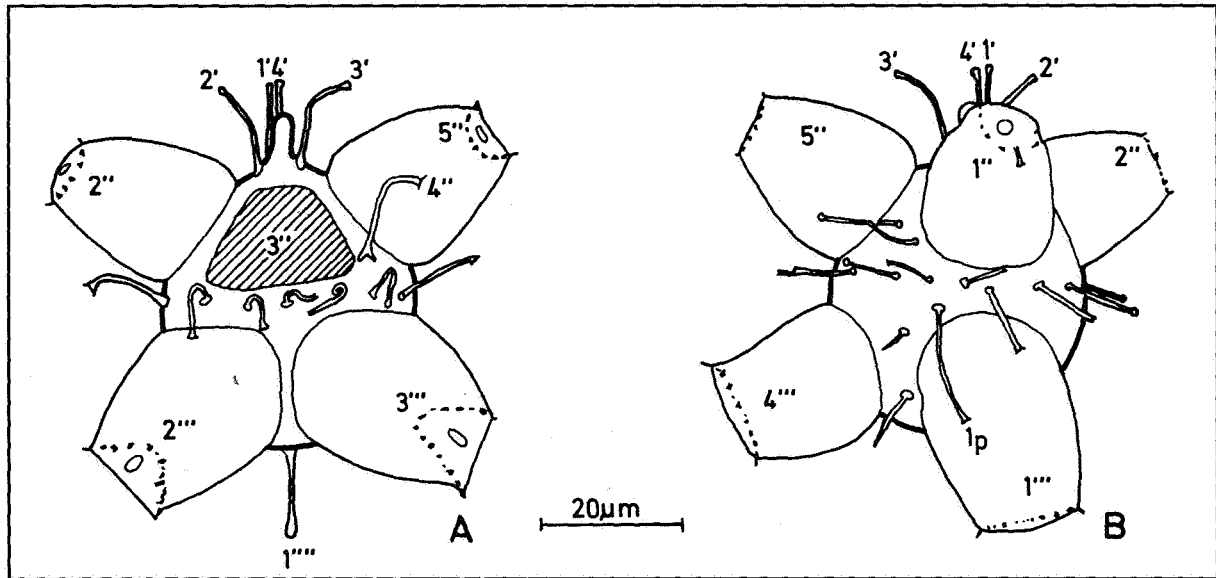
Text-fig. 12: Neoeurysphaeridium glabrum sp. nov., holotype; A, face dorsale en vue externe; B, face ventrale en vue externe.
