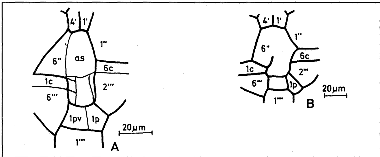
Text-fig. 13: Représentation schématique de l'aire sulcale en vue externe; A, Impagidinium rigidaseptatum sp. nov.; B, Impagidinium scabrosum sp. nov.; lignes épaisses= hauts septes, lignes fines= lignes.
