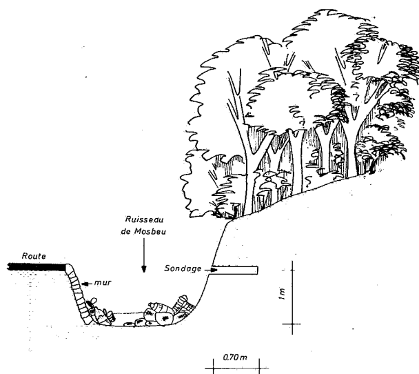
FIG. 8.- Trooz. Position d'un sondage court par rapport à la surface topographique (situation fortement schématisée).
