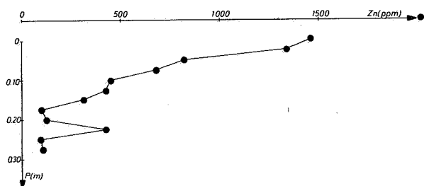
FIG. 7.- Prayon Evolution des teneurs en Zn dans un sondage court.
