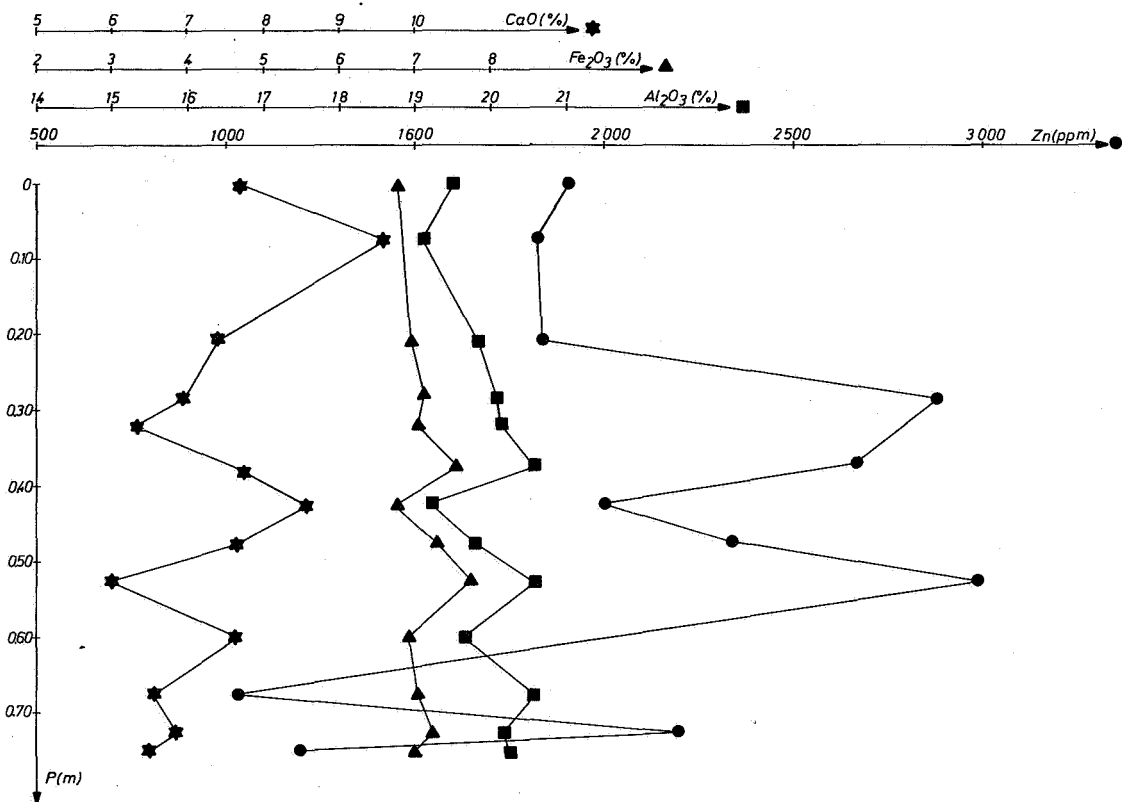
FIG. 9.- Trooz. Evolution des teneurs en CaO, Fe 2 O 3 , Al 2 O 3 et Zn dans un sondage court.
