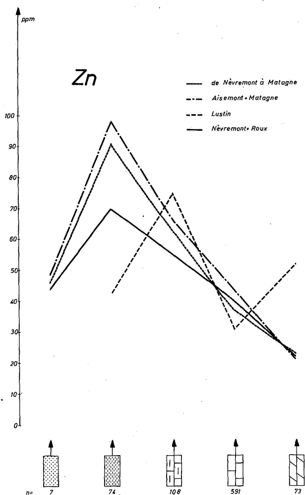
FIG. 19.- Evolution des teneurs en Zn en fonction de la lithologie.
