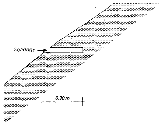
FIG. 6.- Prayon. Position d'un sondage court par rapport à la surface topographique.
