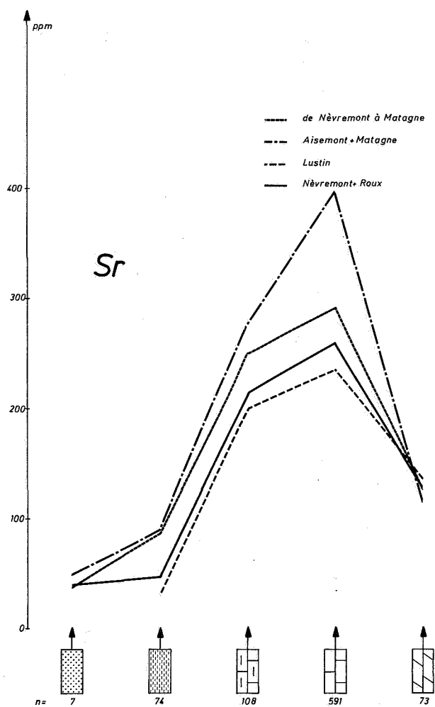
FIG. 16.- Evolution des teneurs en Sr en fonction de la lithologie.
