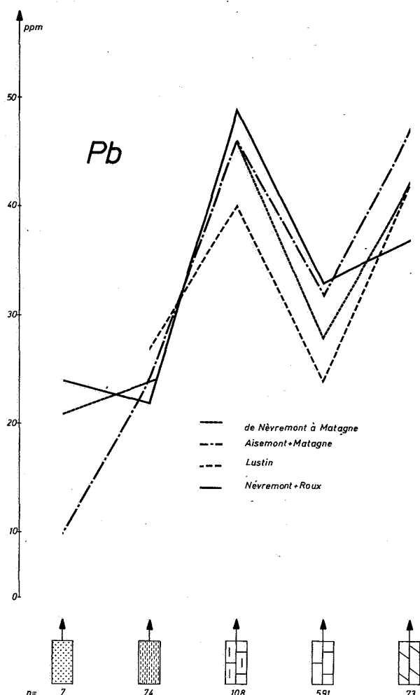
FIG. 17.- Evolution des teneurs en Pb en fonction de la lithologie.
