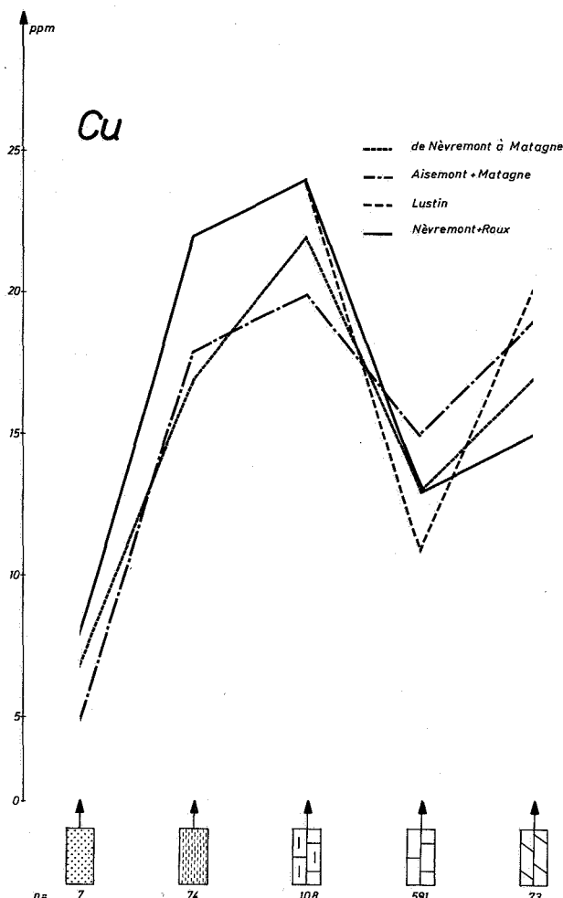
FIG. 18.- Evolution des teneurs en Cu en fonction de la lithologie.
