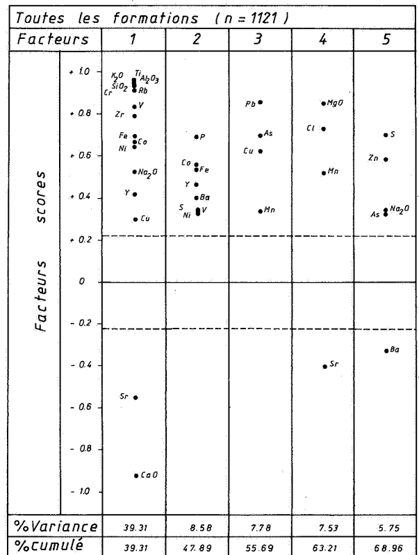
FIG. 20.- Représentation graphique des résultats des analyses factorielles en mode R et en composantes principales appliquées à 4 populations différentes. Les facteurs scores inférieurs au seuil de signification (0.22, Harmann, 1967) n'ont pas été représentés.
