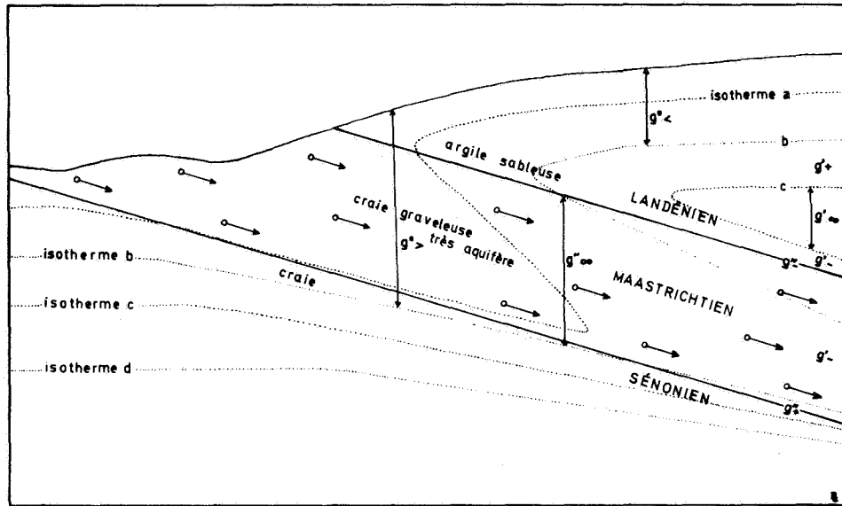
Fig. 1. - Branche froide d'infiltration.
