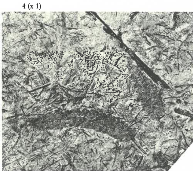
2 - 5 a. Eviostachya Hoegi nov. gen., nov. sp.
