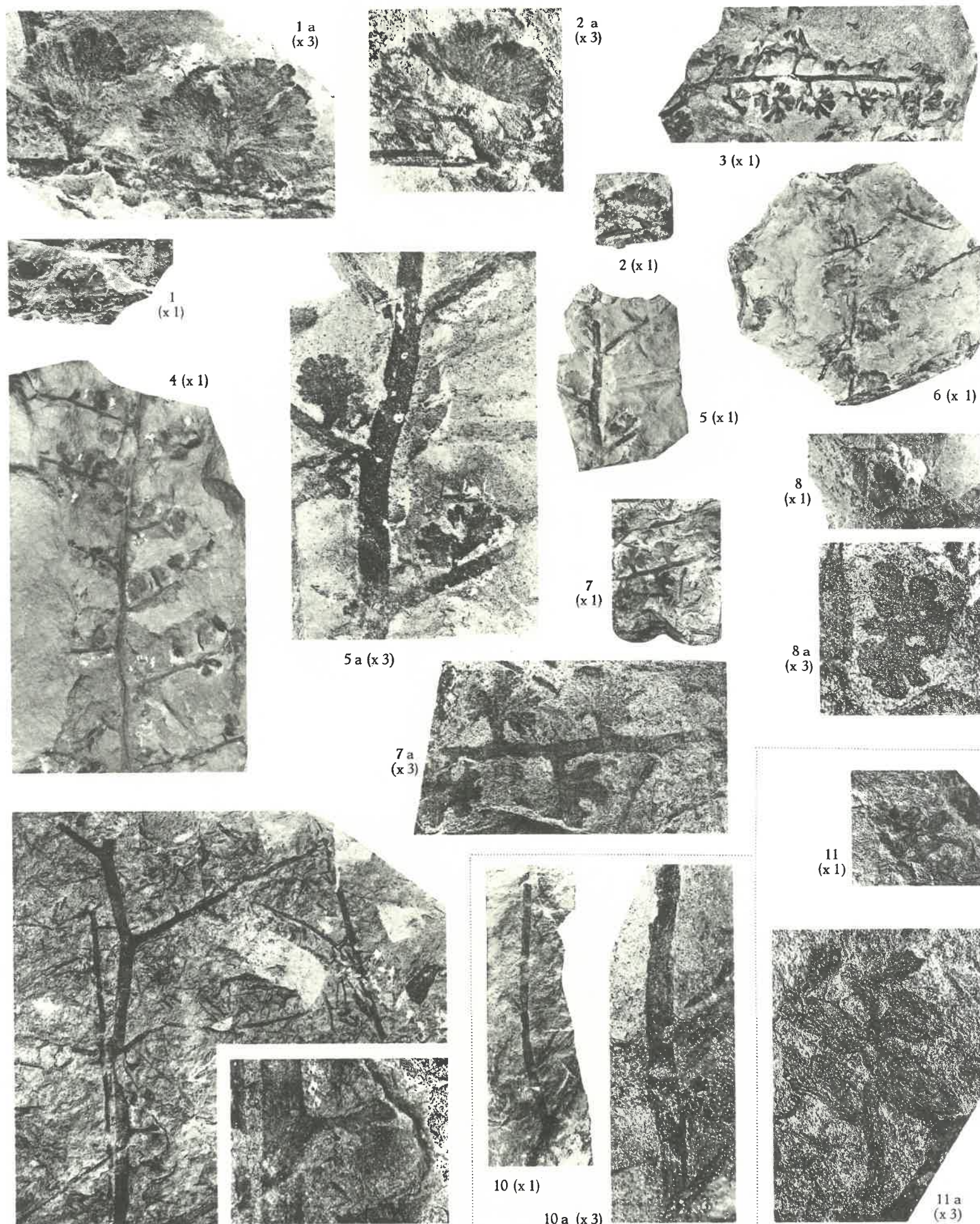
1 - 9 a. Sphenocylopteridium belgicum nov. gen., nov. sp.
