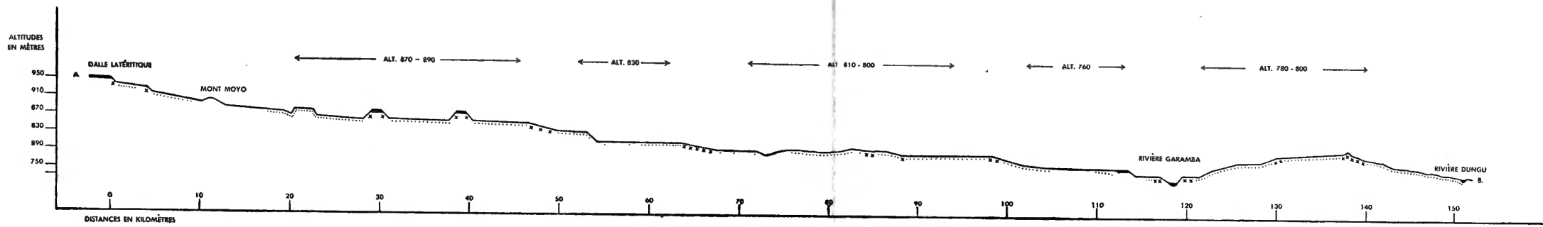
FIG. 1. — Coupe géomorphologique schématique A-B. ..... concrétions latéritiques détritiques; x x x x blocs latéritiques; dalles.
