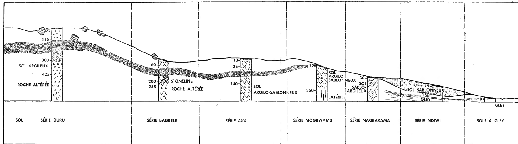
FIG. 6. — Catena des sols III. Région de Bagbélé.
