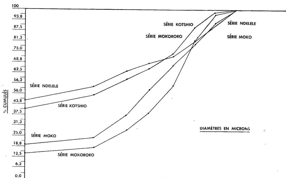
FIG. 9. — Histogrammes granulométriques des sols de la région de Ndelele.
