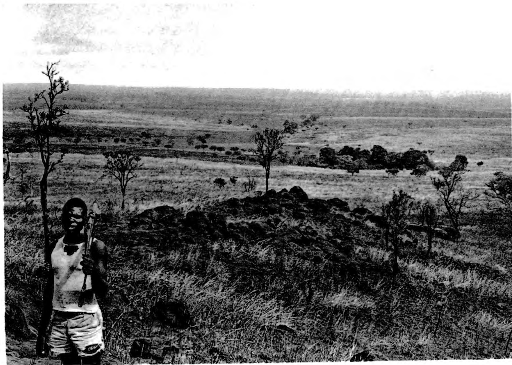
Fig. 1. Surface pénéplanée autour du Mont Bagunda.
