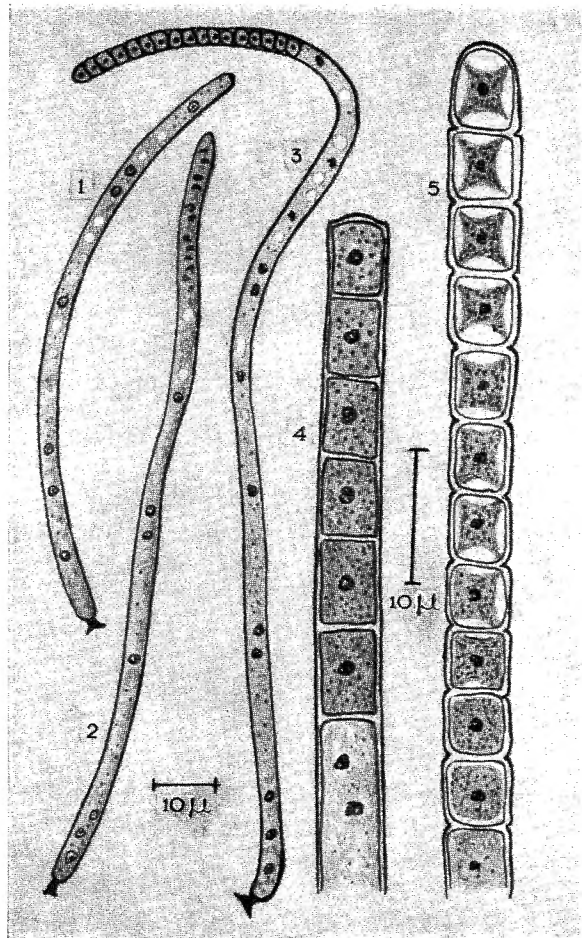
FIG. I. — Eccrinida de Gargilius sp. 1: Filament végétatif; 2: Filament sur le point de donner des éléments reproducteurs; 3: Filament à microarthrocystes; 4 et 5: Différenciation de microarthrocystes à l'extrémité de filaments adultes.
