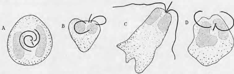
Fig. 7. — Platychrysis pigra . — A, cellule aplatie du film neustique; B, D, cellules s'apprêtant à nager; C, cellule nageant librement. ( \times env. 2500.) D'après CARTER.
