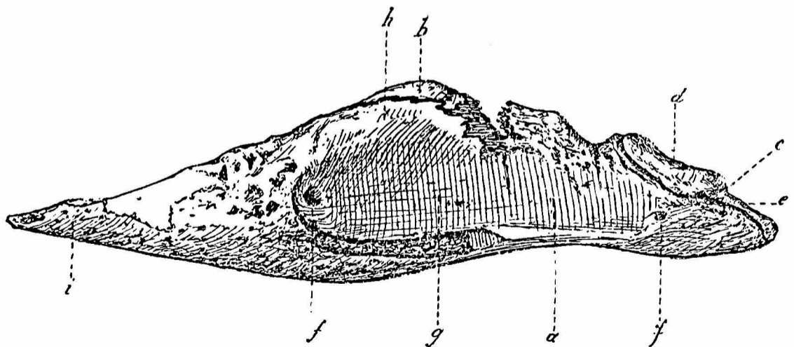
FIG. 2. — Mandibule de la tortue d'Erquellines, vue de profil. Échelle : \frac{2}{3} . Pour la signification des lettres, voir fig. 1.
