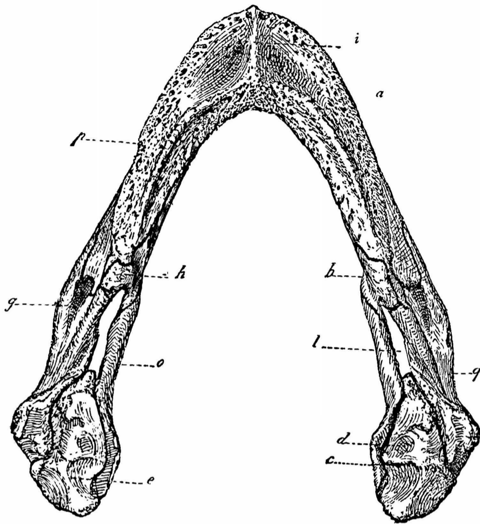
FIG. 3. — Mandibule de Chelonia , vue supérieure.
