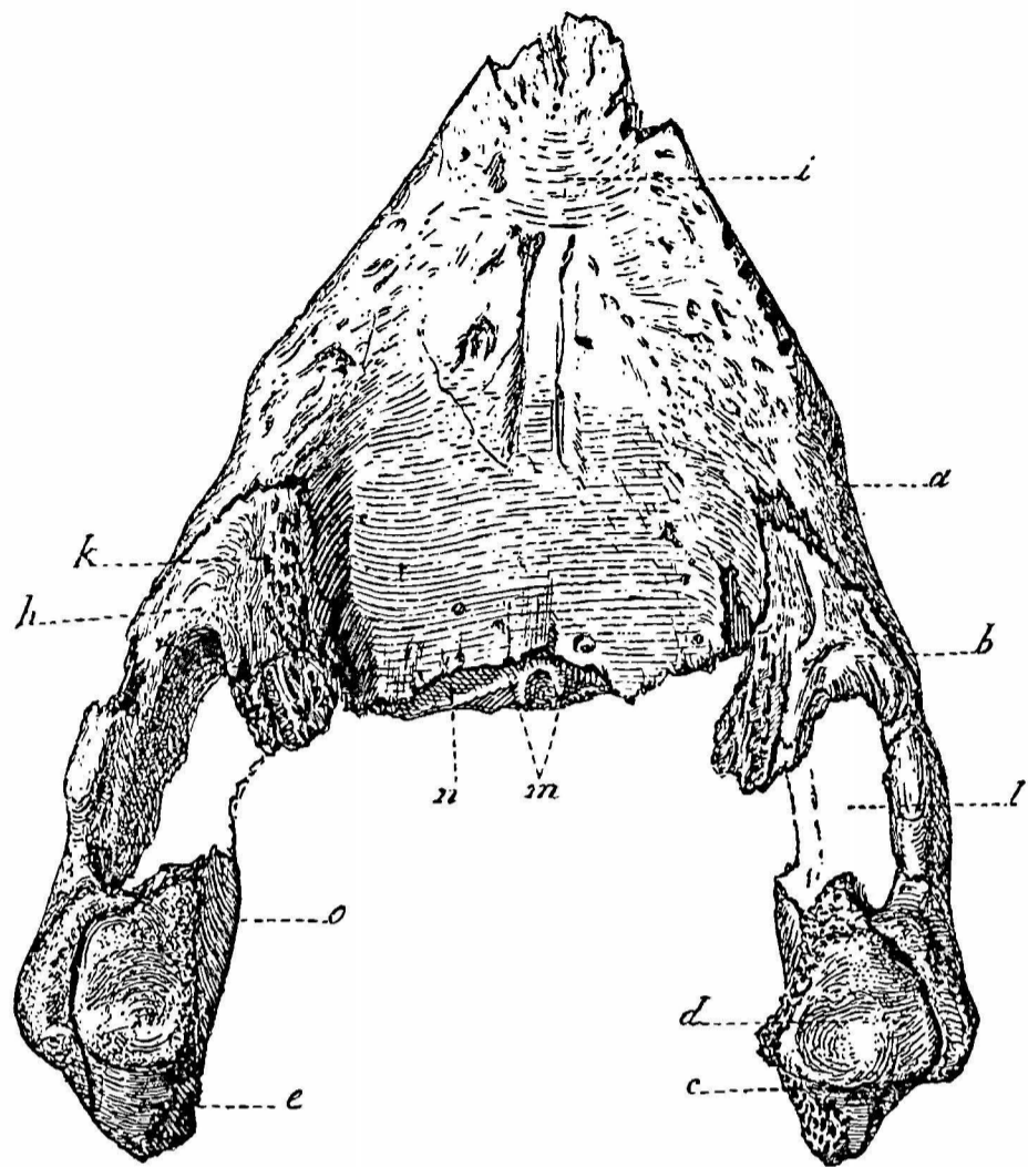
FIG. 1. — Mandibule de la tortue d'Erquellines, vue supérieure. Échelle : \frac{2}{3} .
