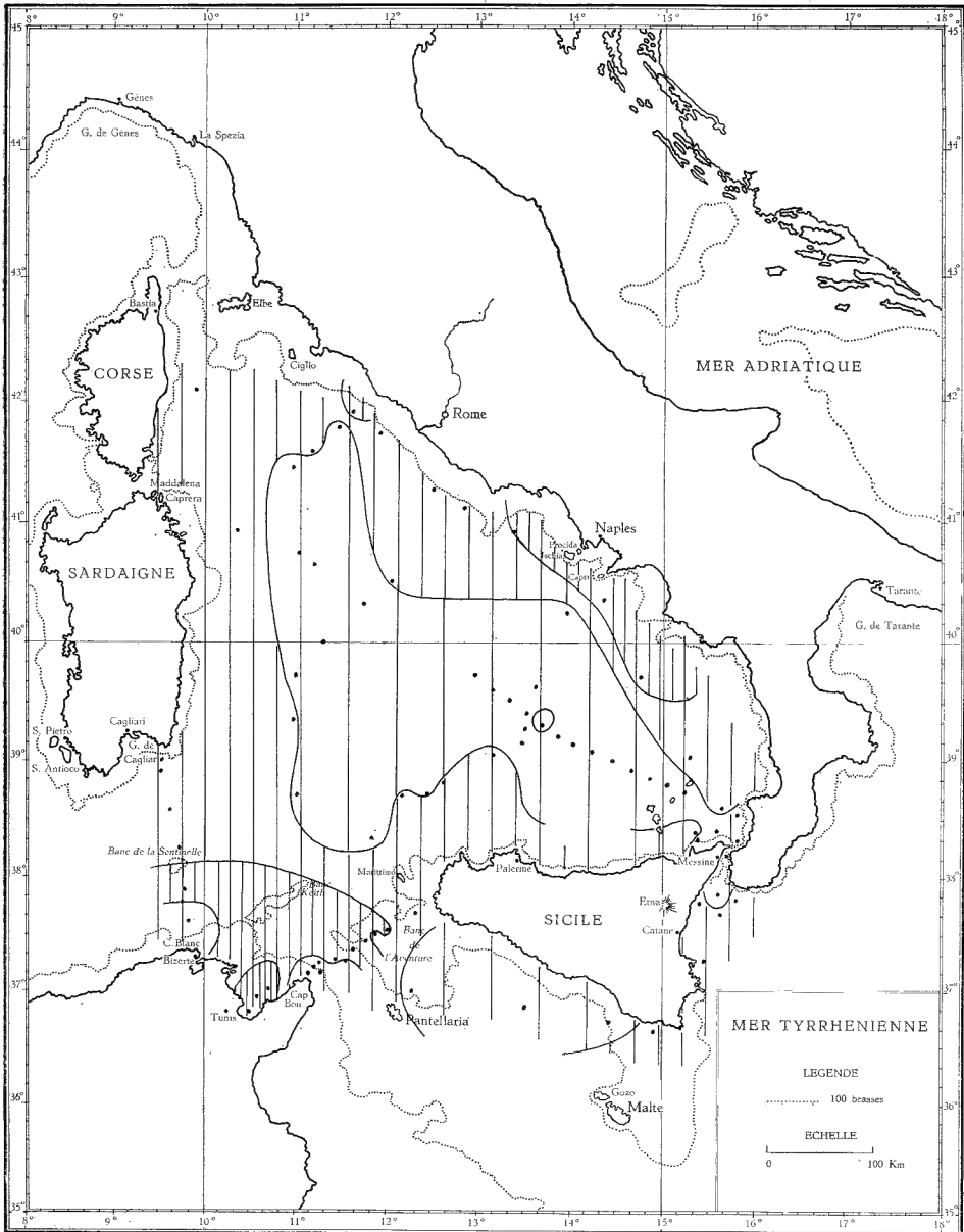
Fig. 11. — Distribution de la chlorophylle a en surface. Les hachures verticales de plus en plus denses signifient : moins de 0,1 \text{ mg/m}^2 de 0,1 à 0,2 \text{ mg/m}^2 de 0,2 à 0,5 \text{ mg/m}^2 plus de 0,5 \text{ mg/m}^2 .
