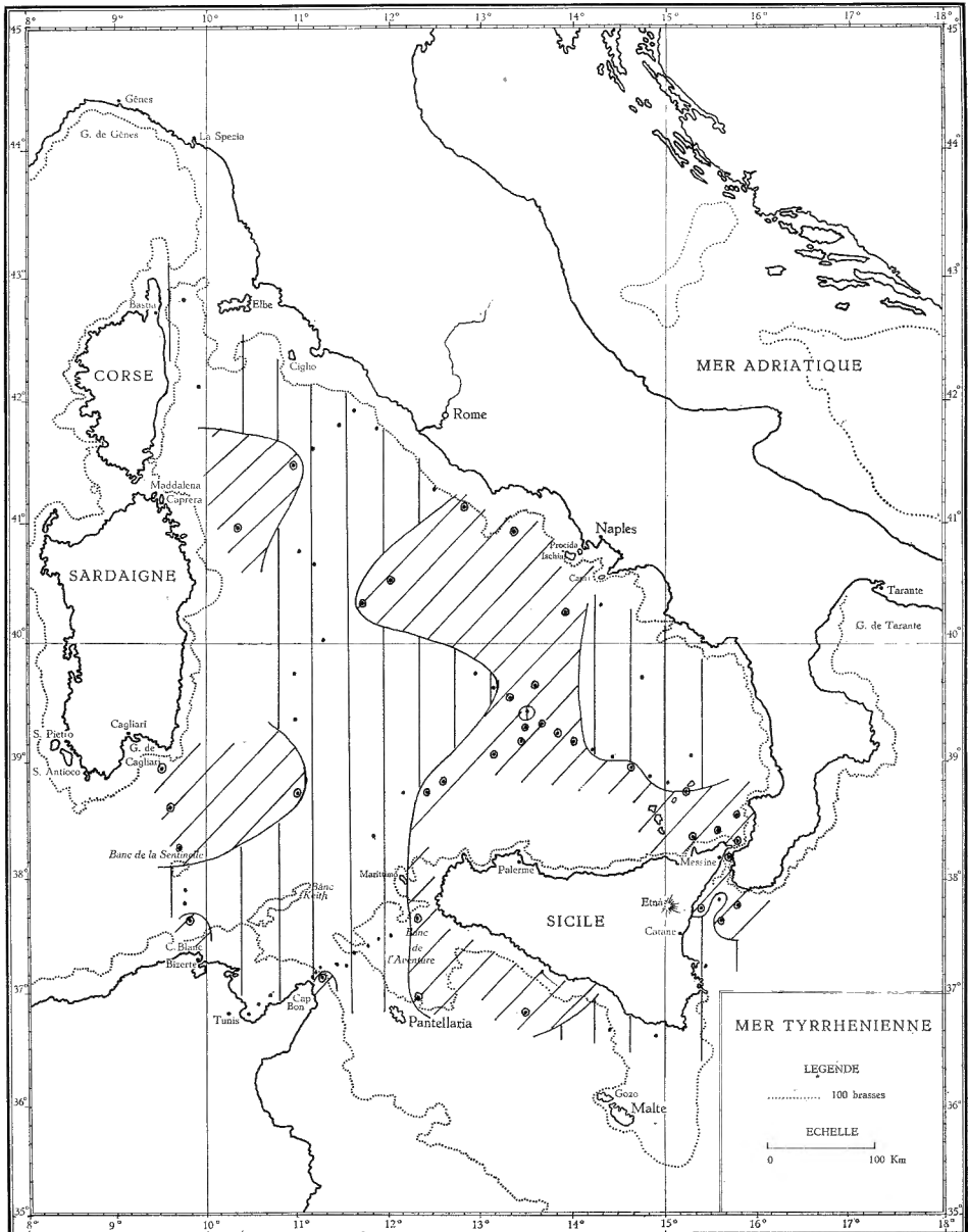
Fig. 13. — Distribution du rapport D_{480}/D_{665} en surface. Les points indiquent les stations d'observation. Les hachures verticales et points simples correspondent aux valeurs inférieures à 4. Les hachures obliques et les points cerclés aux valeurs supérieures à 4.
