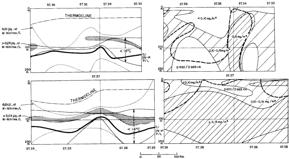
Fig. 15. — Sections verticales se croisant au niveau de la station 27 (ST 27). Voyez la position des stations et la direction des coupes sur la carte de la fig. 1. A gauche : position approximative de la thermocline; distribution des nitrites (la ligne en points représente le niveau de 0,01 \mu\text{g-at. N-NO}_2/\text{l} , la partie pointillée, les concentrations supérieures à 0,03 \mu\text{g-at. N-NO}_2/\text{l} ) et distribution des phosphates (la ligne en gras représente le niveau 0,1 \mu\text{g-at. P-PO}_4/\text{l} de la concentration en phosphates, plus élevée vers le bas). Les limites supérieure et inférieure de la couche d'eau à moins de 14^\circ\text{C} sont indiquées par deux lignes simples. A droite, distribution de la chlorophylle a (en blanc, moins de 0,10 \text{ mg/m}^3 ; en hachures espacées, 0,10-0,15 \text{ mg/m}^3 ; en hachures plus denses, plus de 0,15 \text{ mg/m}^3 ) et de l'indice D_{430}/D_{665} (la ligne à traits discontinus représente les valeurs de l'indice inférieures à 4 vers le bas et supérieures à 4 vers le haut).
