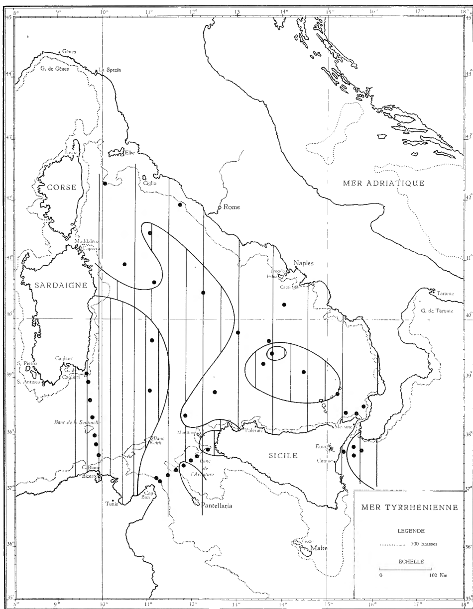
Fig. 8. — Distribution du P-phosphate à 100 m de profondeur aux différentes stations. Les hachures verticales de plus en plus denses signifient :
