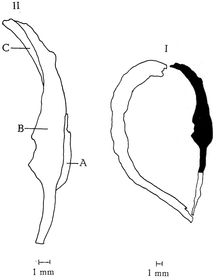
Fig. 10. — Schizophoria striatula (E. SCHLOTHEIM). I : lame mince dans le plan de symétrie bilatérale. La partie noire correspond au dessin II et à la Fig. 4, Pl. II. II : détail de I. — A : fibrotest. — B : prismotest. — C : callotest.
