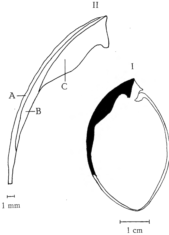
Fig. 12. — Terebratula maxima E. CHARLESWORTH emend. H. MUIR-WOOD. I : profil de coquille. La partie noire correspond au dessin II et à la Fig. I, Pl. II. II : détail de I. — A : fibrotest. — B : prismotest. — C : callotest.
