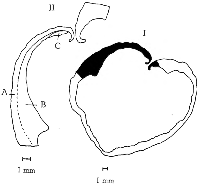
Fig. 1. — Platystrophia ponderosa auburnensis A. F. FOERSTE. I : lame mince dans le plan de symétrie bilatérale. La partie noire correspond au dessin II et à la Fig. 1, Pl. I. II : détail de I. — A : fibrotest. — B : prismotest. — C : callotest.
