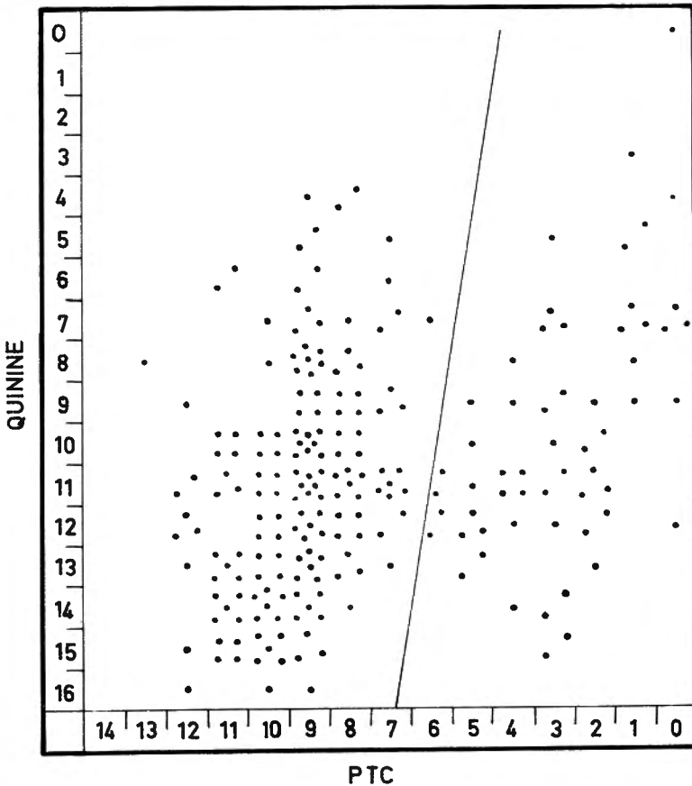
Fig. 5. — Corrélation entre les seuils de sensibilité à la P.T.C. et à la quinine chez 225 hommes et droite de meilleure séparation entre goûteurs et non-goûteurs.
