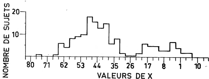
Fig. 11. — Histogramme des fréquences absolues des valeurs de la fonction X chez 158 hommes de 18 à 28 ans.
