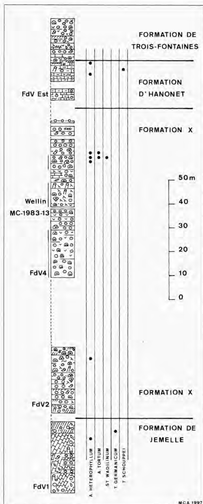
Fig. 4 – Log schématique du Fond des Vaux à Wellin avec la distribution de quelques Rugueux. (Pour la légende des signes conventionnels, voir fig. 3).
