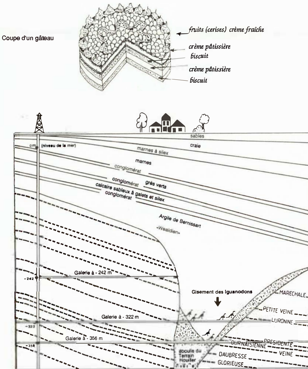
Coupe du puits Sainte Barbe
