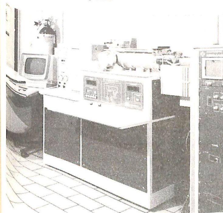
Figure 8 Spectrométrie de masse couplée à la chromatographie en phase gazeuse
