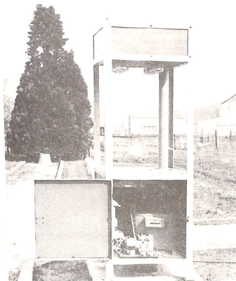
Figure 12 Cabine pour études poussières
