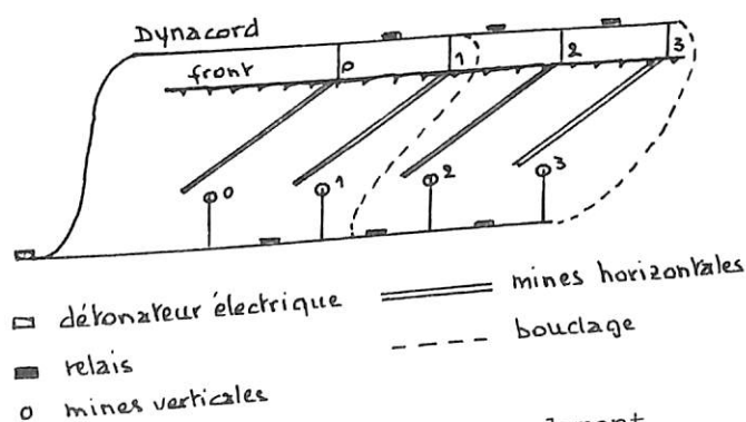
Fig. 2 - Schéma de raccordement
