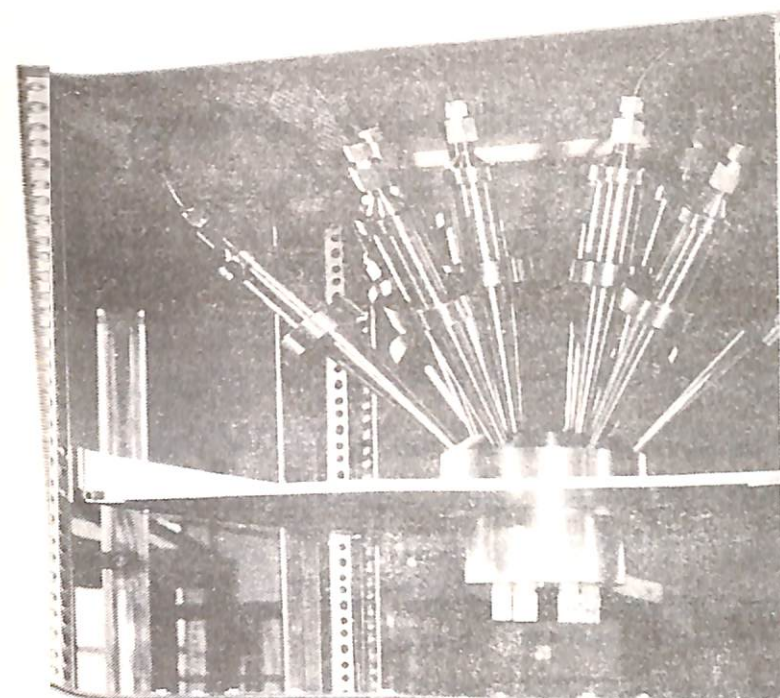
Figure 10 Système de prélèvement mis au point à l'INIEX
