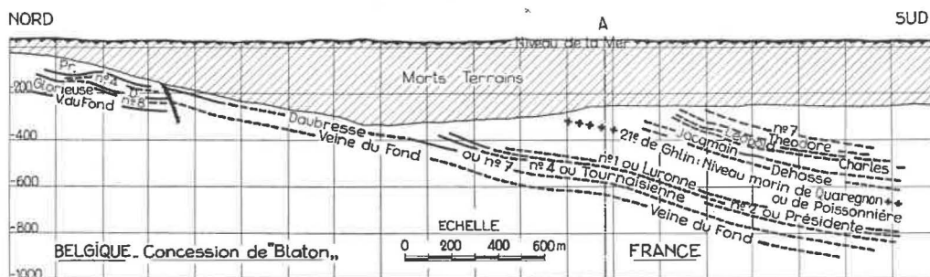
Coupe schématique Nord-Sud passant par le point A de la carte.
