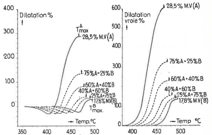
Fig. 34. — Courbes dilatométriques (Audibert-Arnud) et dilatations vraies calculées de mélanges binaires.
