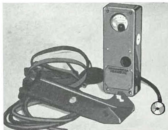
Fig. 17. — Grisomètre « Verneuil » et ses accessoires (plaque support et poire de prélèvement).
