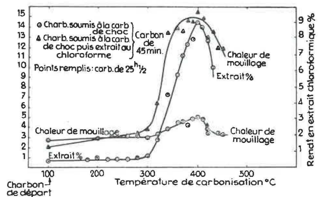
Fig. 40. — Rendements en extrait et chaleur de mouillage de charbon carbonisé, avant et après extraction au chloroforme.
