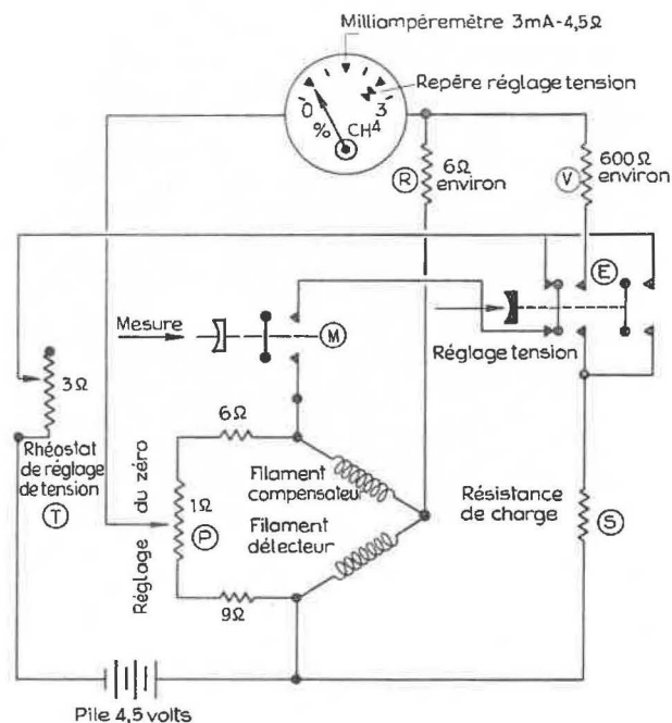
Le commutateur E "réglage de tension" est lié à la commande du rhéostat de réglage de tension
