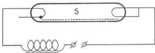
Fig. 11. — Lampe à allumage instantané sans préchauffage des électrodes avec bande intérieure conductrice S.
