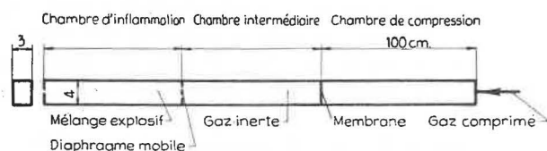
Fig. 15. — Tube de choc.
