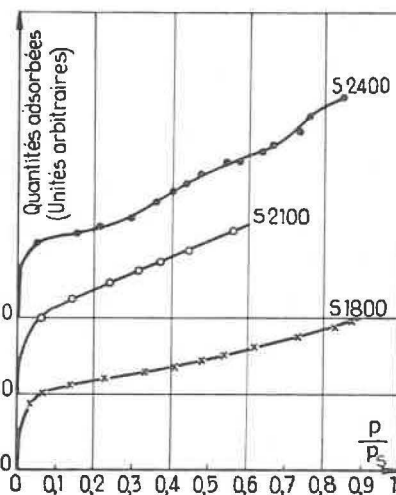
Fig. 49. — Isothermes d'adsorption de méthane à - 196° C sur charbons de polyvinylidène.
