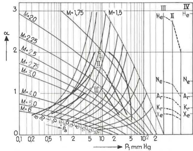
Fig. 13. — Graphique \alpha - p_1 de l'afflux d'un gaz biatomique à 1 atm contre un remplissage de gaz rare à basse pression.
