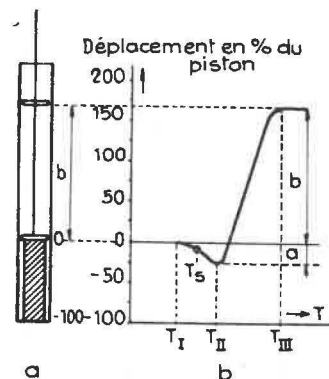
Fig. 31. — Courbe dilatométrique du dilatomètre Audibert-Arnu.
