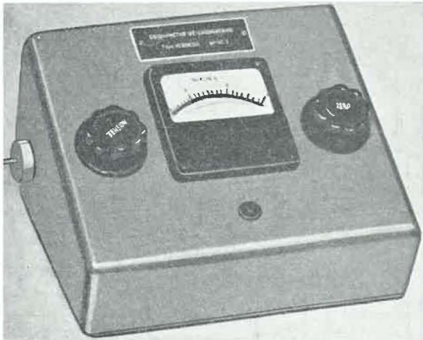
Fig. 18. — Grisomètre « Vernuil - Laboratoire ».
