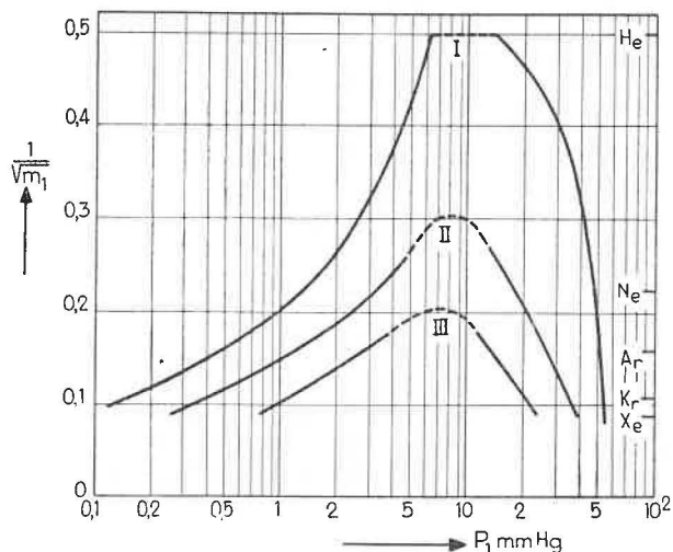
Fig. 14. — Limites d'inflammation dynamique dans un graphique comportant comme coordonnées p_1 et 1/\sqrt{m_1}
