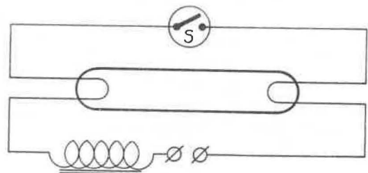
Fig. 10. — Lampe à fluorescence montée normalement avec bobine de choc utilisée comme ballast et starter S.
