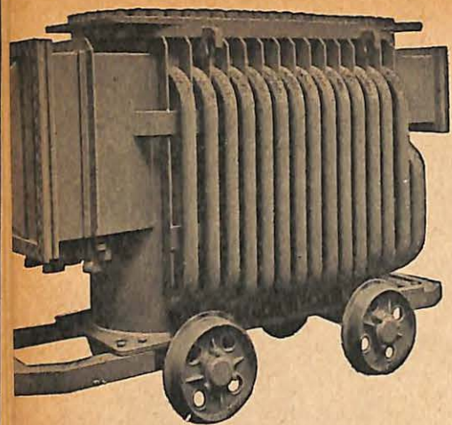
Transformateur anti-déflagrant pour mine grésouteuse.
