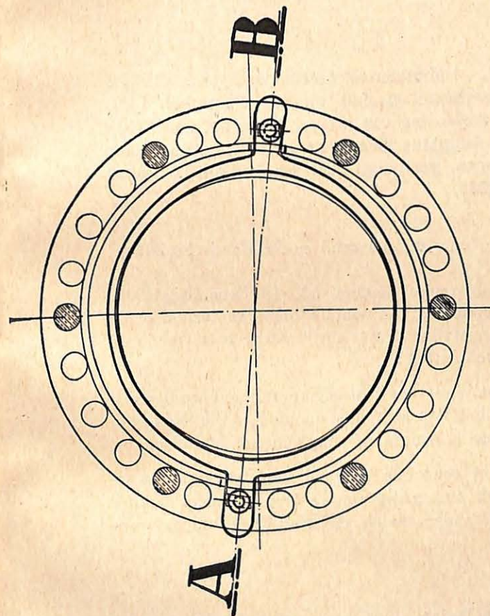
Teekening 4 : Toegelaten schikking voor de bestaande lampen : vastmaking door een veer-ring.
