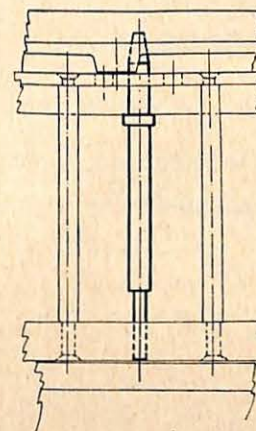
TEEKEN. 1. — Tusschen twee beschermingsstaven geplaatste sluitingsgrendel.
