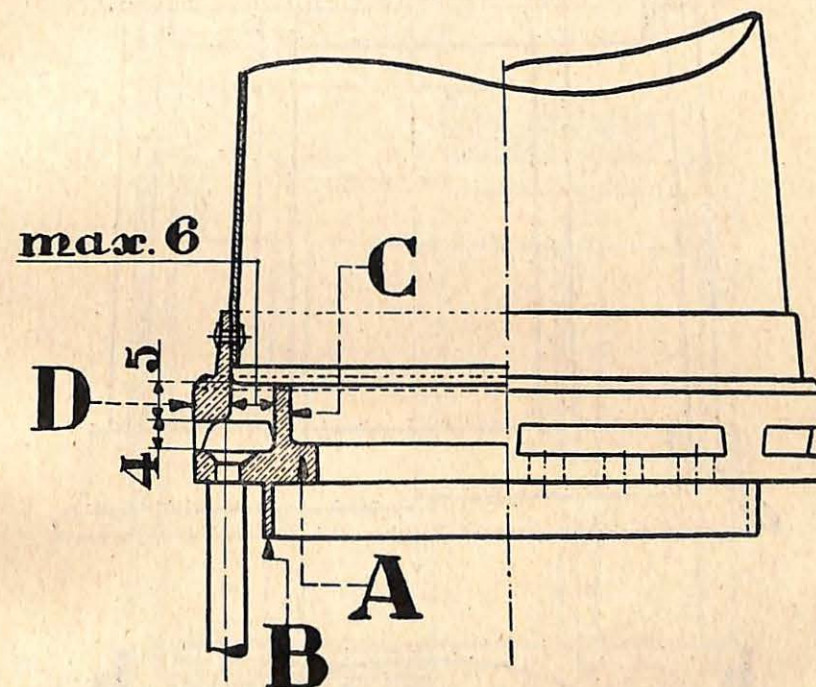
Teekening 1 : Schikking van het onafzetbaar omhulsel.
