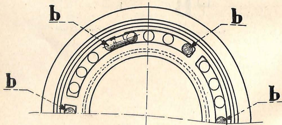
Teekening 2 : Toegelaten schikking voor de bestaande lampen : vastmaking door een geplooid staaf.
