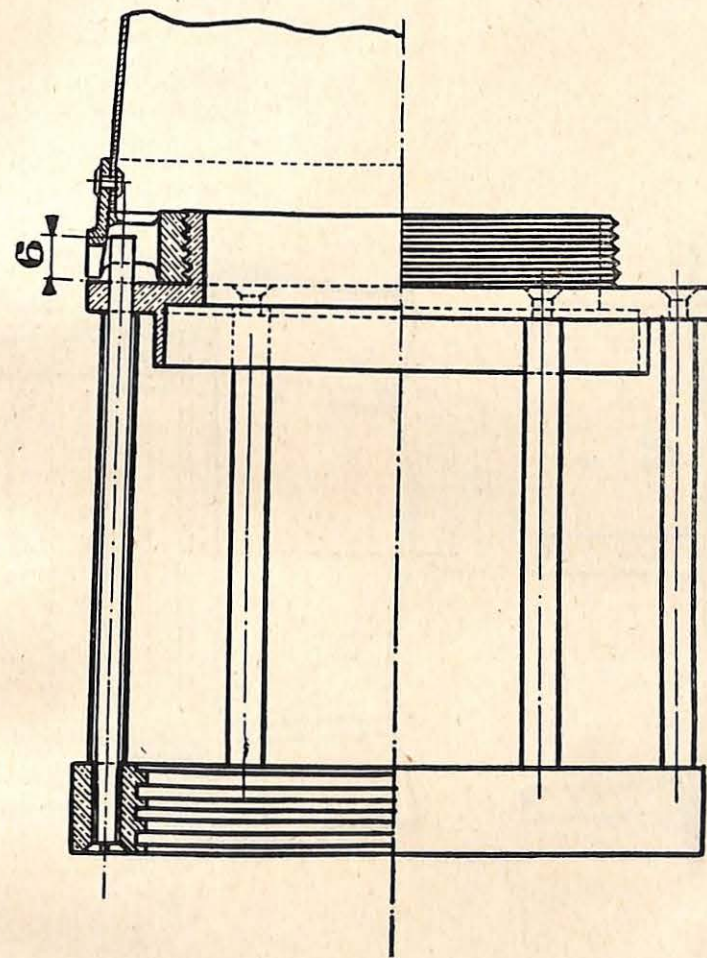
Teekening 3 : Toegelaten schikking voor de bestaande lampen : vastmaking door een geschroefde en door een vrij draaiend buisje omringde slang.
