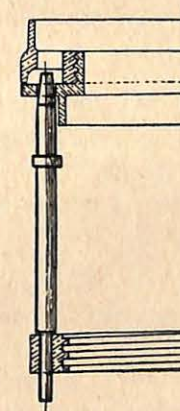
TEEKEN. 3. — Schikking van den grendel in de uiteengezette armatuur alleen, de ontschroefing van het omhulsel toelaten.
