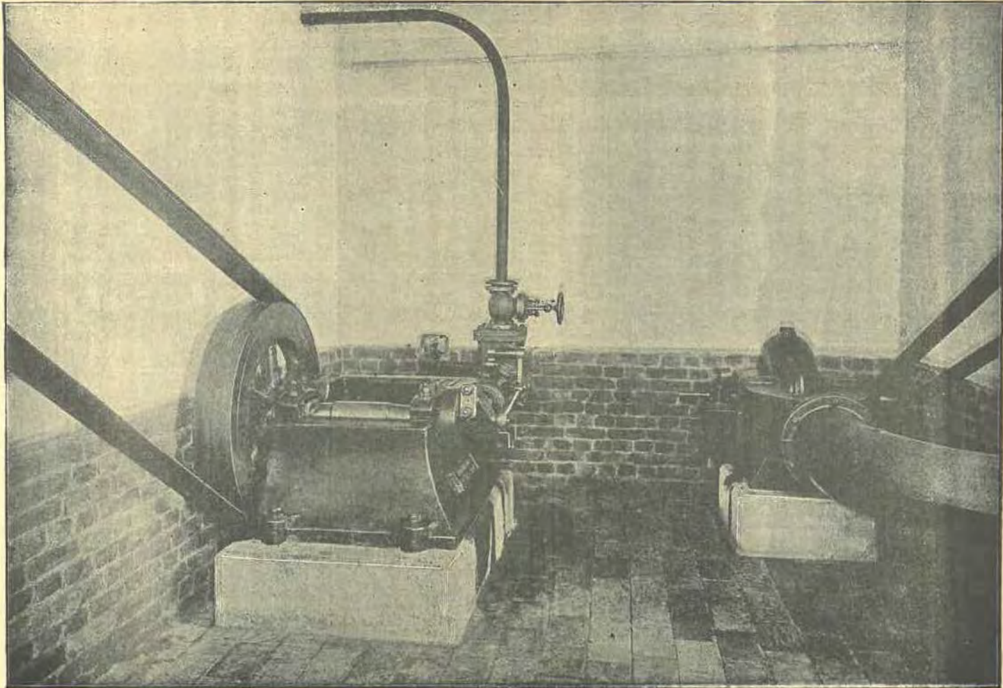
FIG. 30 — Vue du moteur et du ventilateur-aspirateur.
