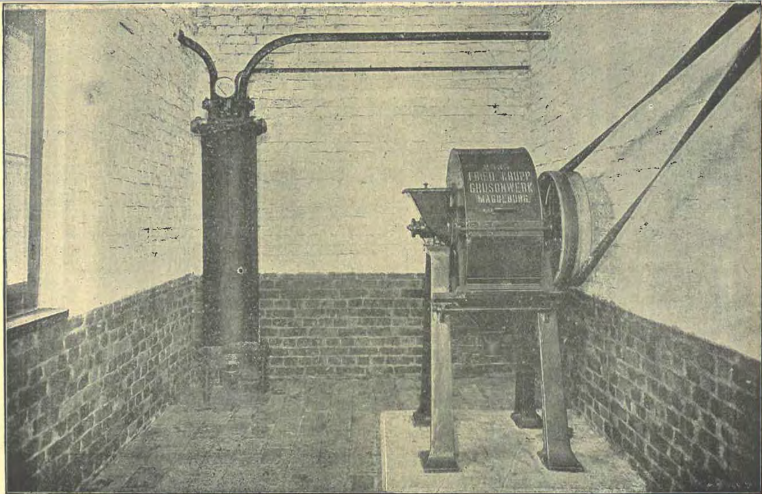
FIG. 32. — Vue du broyeur à boulets et du sécheur de vapeur.
