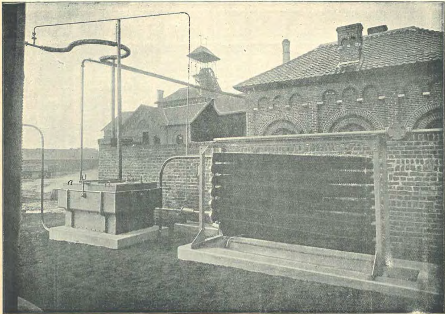
FIG. 19. — Vue de l'aspirateur, du condenseur et de l'épurateur.
