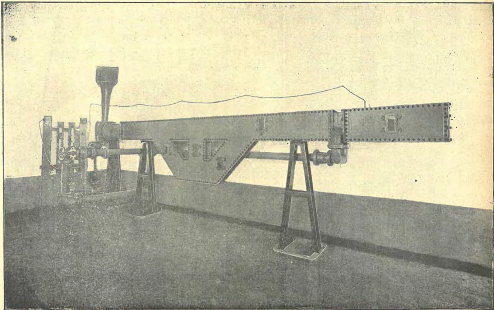
FIG. 7. — Appareil pour l'essai des lampes de sûreté.
