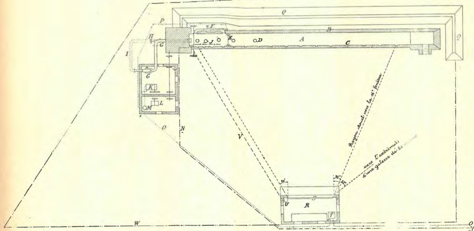
FIG. 28. — Dispositif d'ensemble du siège d'essai des explosifs.
