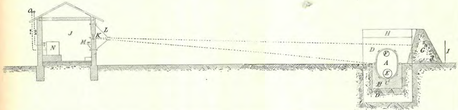
FIG. 29. — Coupe en travers du siège d'essai des explosifs.
