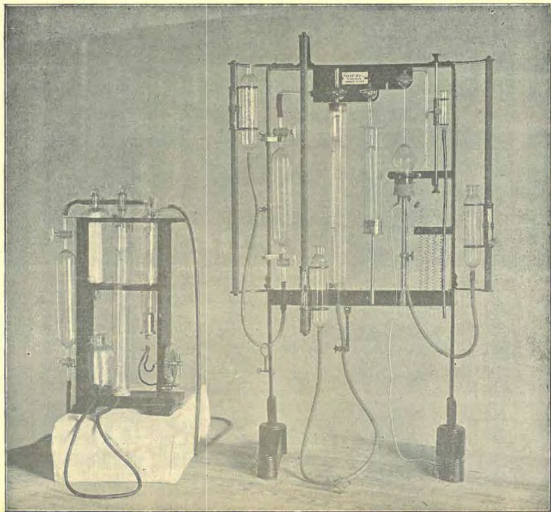
FIG. 27 — Vue des grisoumètres de Mertens et de Schondorf. GALLADÉ, phot., Mons
