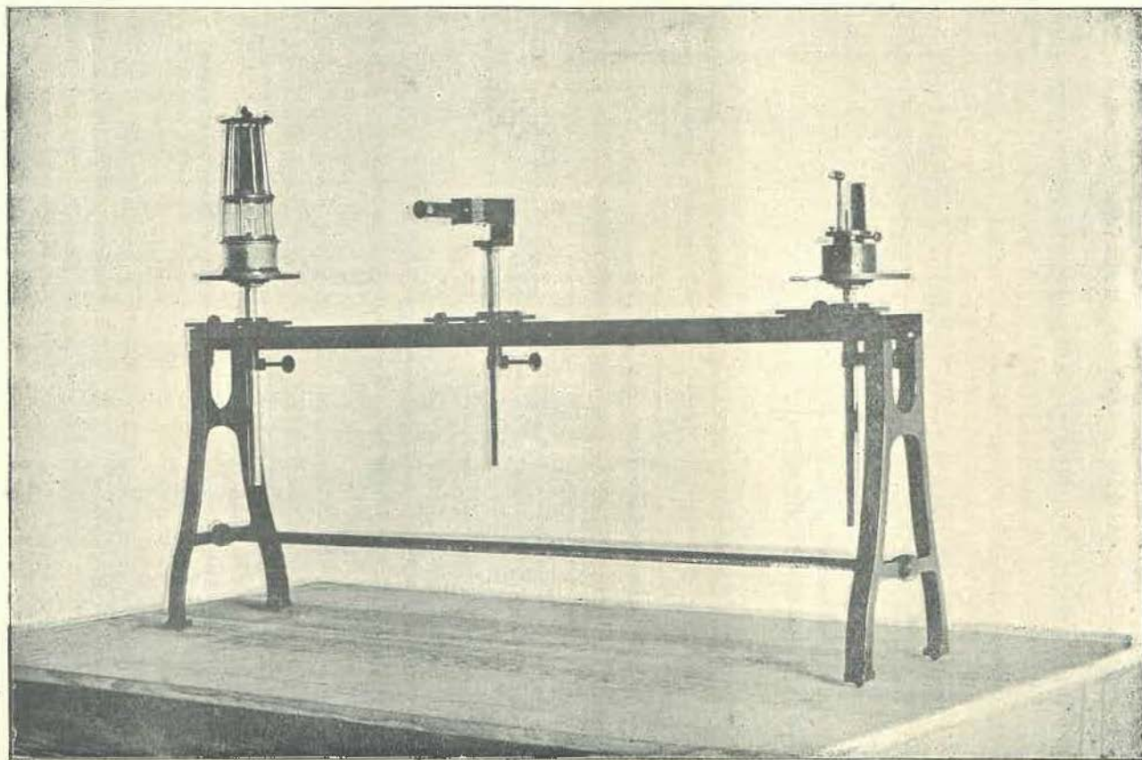
FIG. 26. — Vue du banc photométrique.
