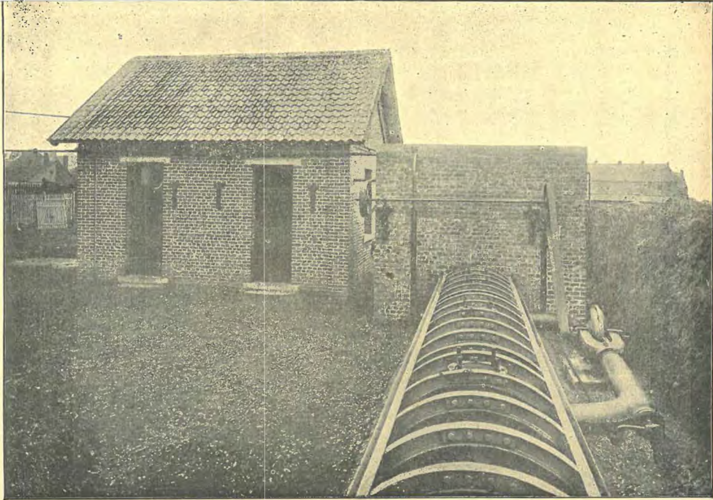
FIG. 6. — Vue de la galerie d'essai des explosifs et du ventilateur mélangeur.
