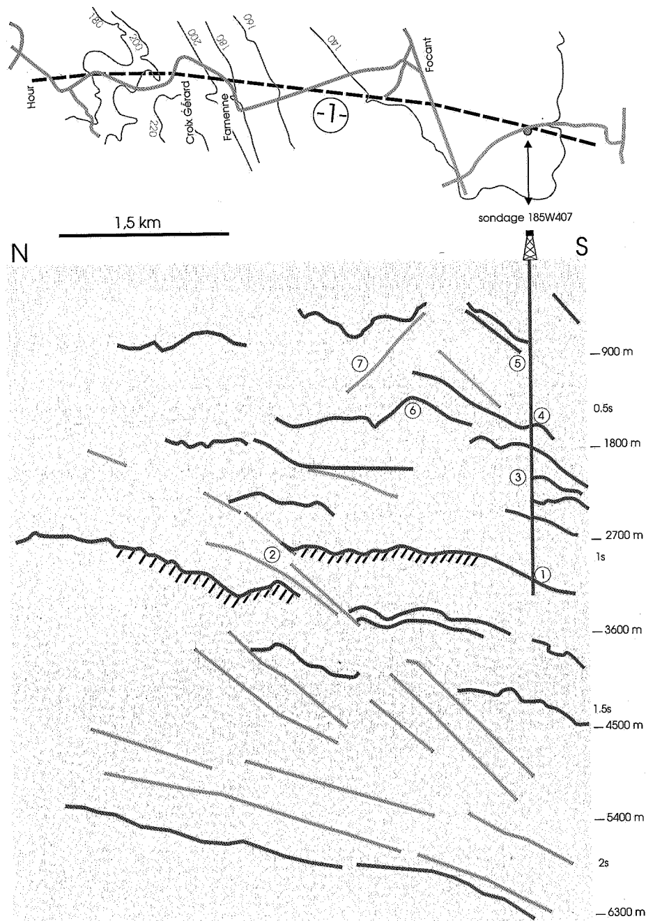
Figure 9. Localisation et extrait de la section sismique 1, effectuée en 1976 et passant par le sondage 185W407 de Focant. «1» à «7»: marqueurs sélectionnés (explications dans le texte).
