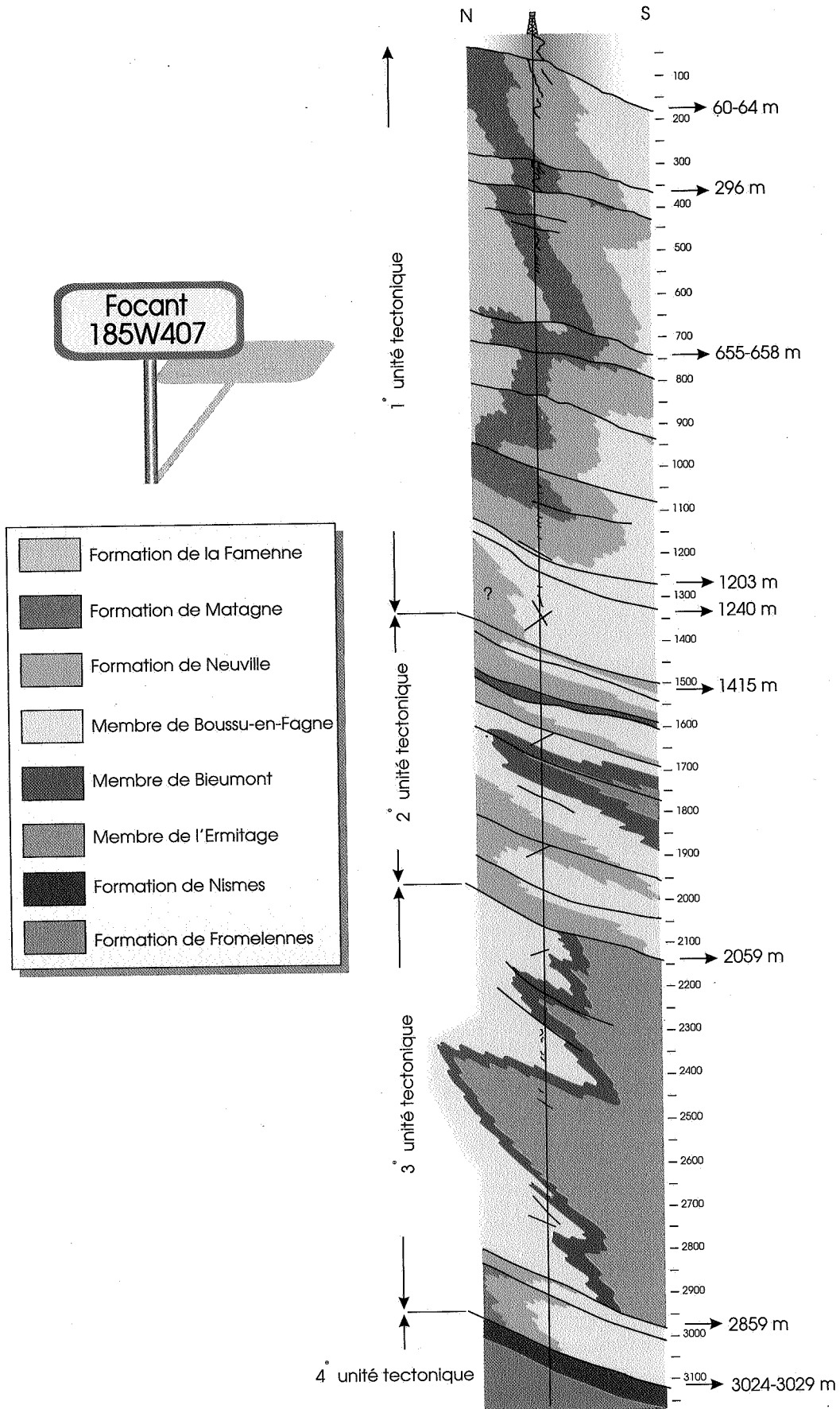
Figure 8. Coupe synthétique globale du sondage 185W407 de Focant.
