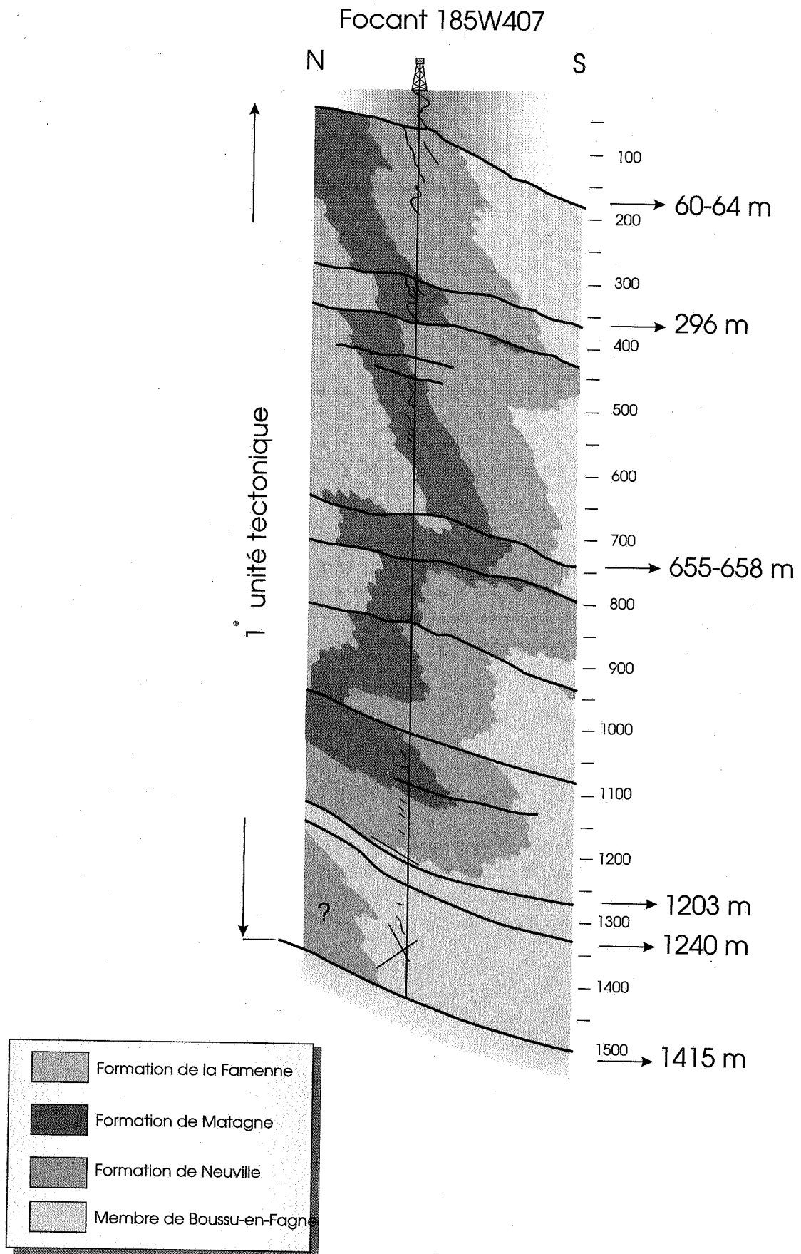
Figure 6. Coupe synthétique du sondage 185W407 de Focant (première unité tectonique).
