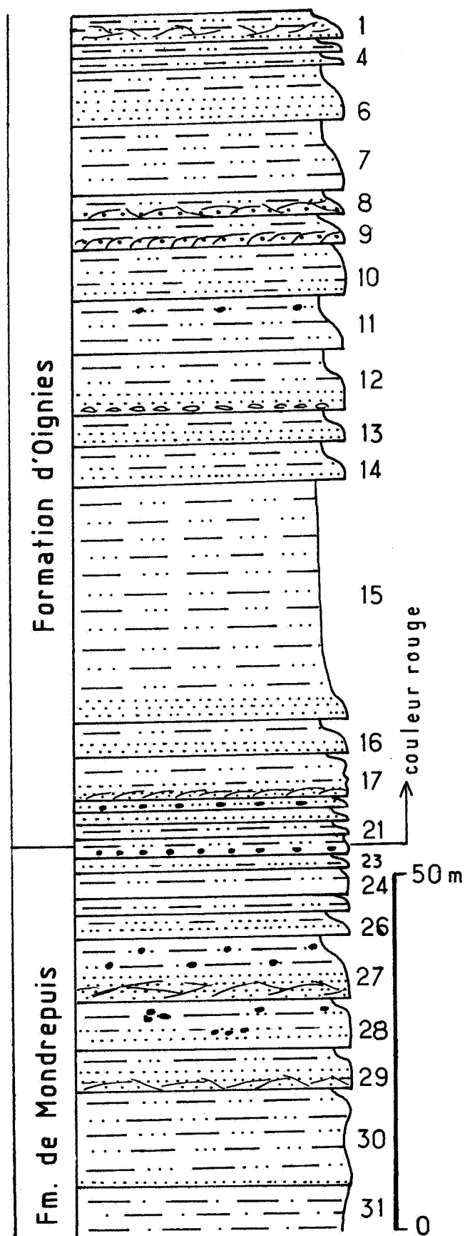
Figure MON/OIG-2. Colonne stratigraphique du sommet de la Formation de Mondrepuis et de la partie inférieure de la Formation d'Oignies.
