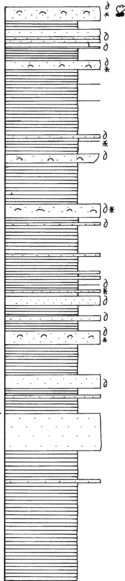
Figure VIL-2. Colonne stratigraphique du sommet de la Formation de Mirwart et de la base de la Formation de Villé à Villé (stratotype de la Formation de Villé).
