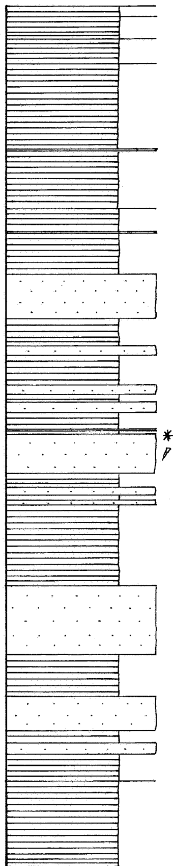
Figure VIL-2. Colonne stratigraphique du sommet de la Formation de Mirwart et de la base de la Formation de Villé à Villé (stratotype de la Formation de Villé).
