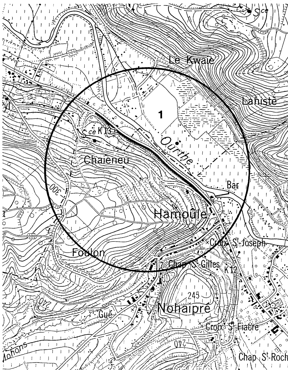
Figure HAM-1. Extrait de la carte topographique IGN n° 55/5 à 1/10 000 Hotton avec indication du stratotype de la Formation de Hampeau.
