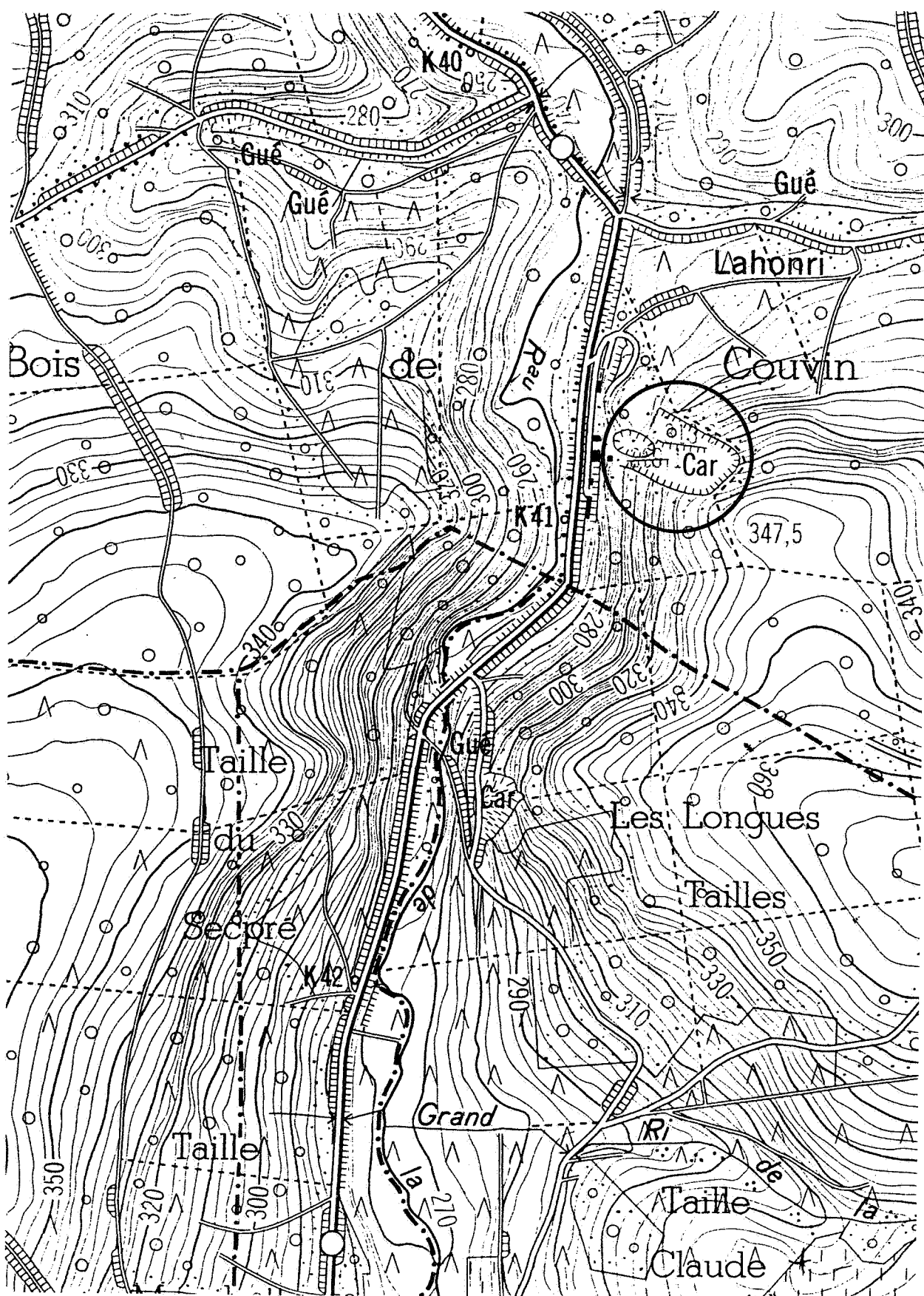
Figure FEP-1. Extrait de la carte topographique IGN n° 62/4 à 1/10 000 Cul-des-Sarts avec indication du stratotype de la Formation de Fépín.
