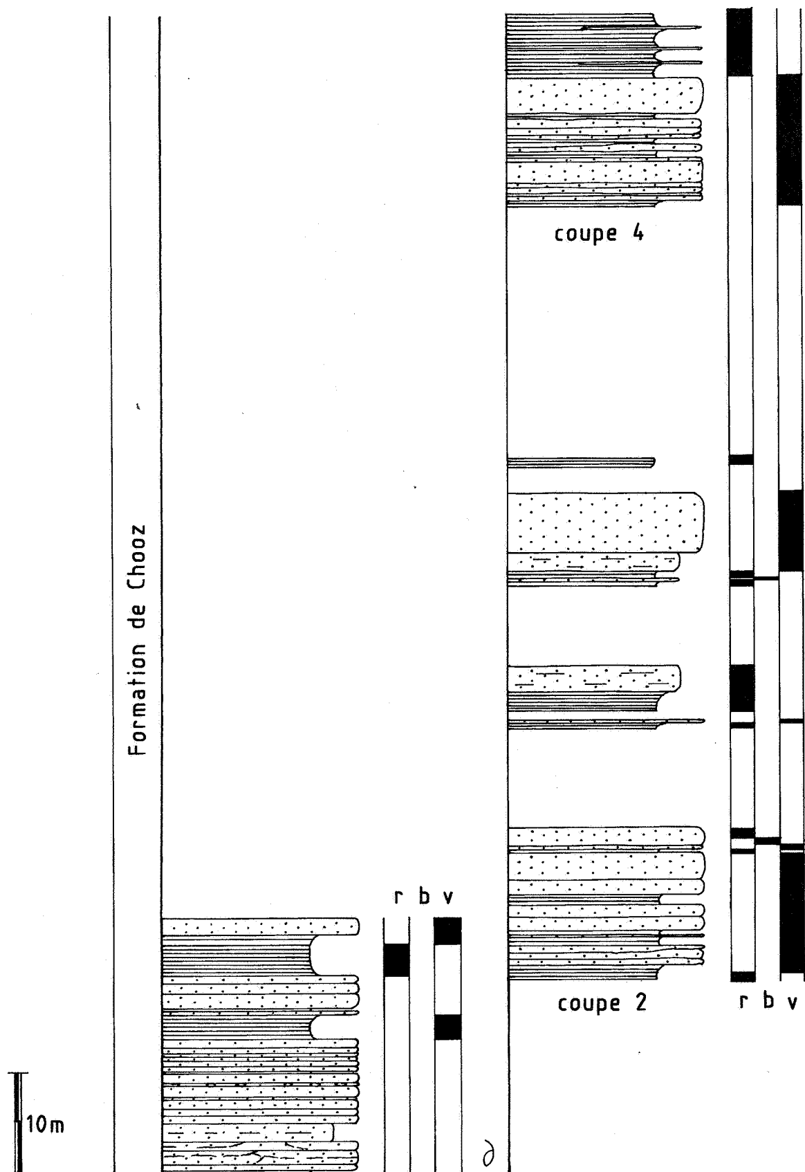
Figure VIR/CHO-6. Colonnes stratigraphiques de la Formation de Chooz à la carrière du Mont Vireux, le long du chemin d'accès à la carrière (coupe 2) et au lieu-dit «Les Rouges Terres» (coupe 4).
