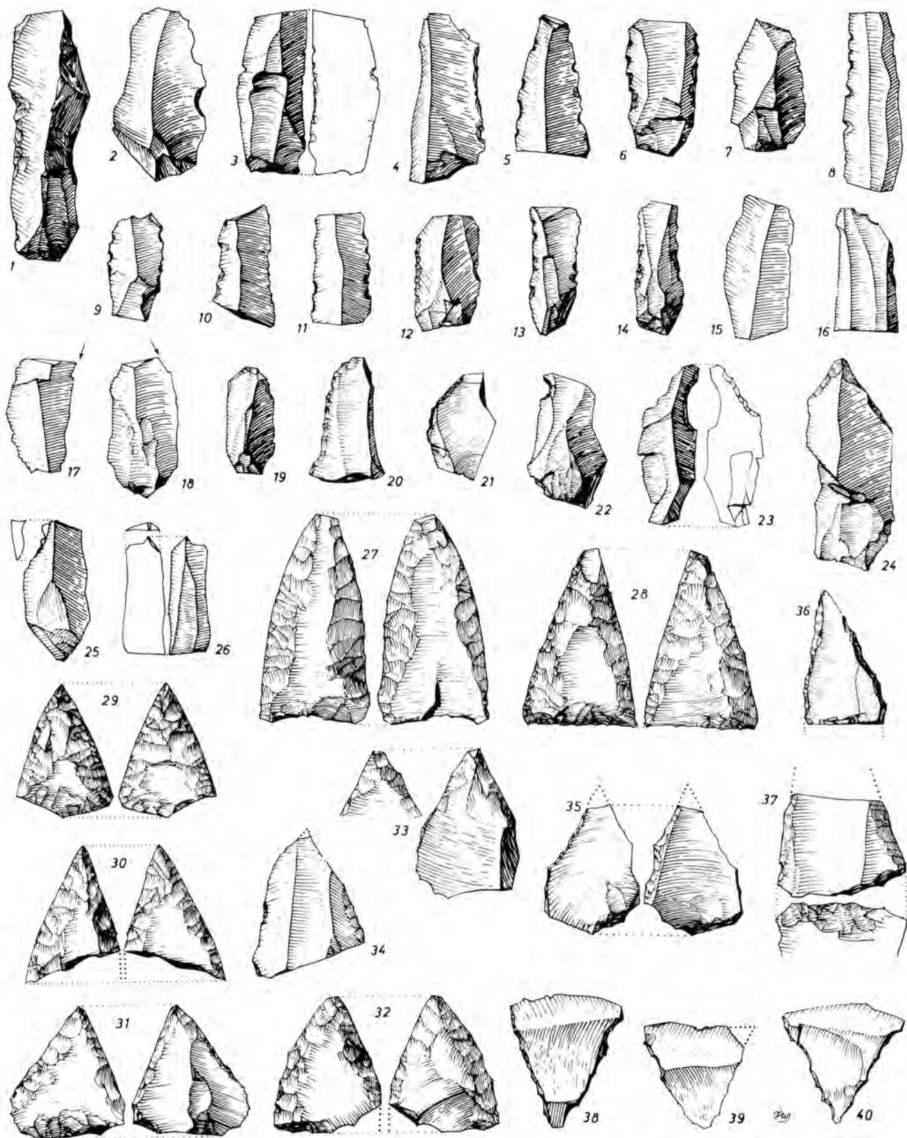
FIG. 31. — Outils sur lamelle et pointes de flèche 1) Retouche normale; (H7-T). 2) Retouche denticulée; (déblais). 3) Id.; (G4+2). 4) Id.; (F4-T-18). 5) Id.; (G4). 6) Id.; (G5-T). 7) Id.; (G6-T). 8) Id.; (G4-20). 9) Id.; (F4-T). 10) Id.; (G4). 11) Id.; (G4). 12) Id.; (G4). 13) Id.; (G6-T). 14) Retouche denticulée; (F4-T). 15) Retouche faible; [G5-T]. 16) Id.; (H7-T). 17) Burin diminutif sur cassure; (18-S). 18) Id.; (Niv. inf.). 19) Troncature convexe; (G5-T). 20) Retouche et cassure; (H6-S). 21) Id.; (A2-10). 22) Id.; (Niv. inf.). 23) Retouche et encoche alternes; (H7-T). 24) Lamelle appointée; (L7-S). 25) cf. Microburin; (18-S). 26) Id.; (sans indication). 27) Pointe de flèche du sous-type 21A, à retouche bifaciale et supérieure à 3 cm; ébréchure de pointe; specimen (a); (H7-T-37). 28) Id.; specimen (b); (18-S). 29) Pointe de flèche du sous-type 21B, à retouche bifaciale et inférieure à 3 cm; specimen (e), complet; (G5-T-5). 30)
