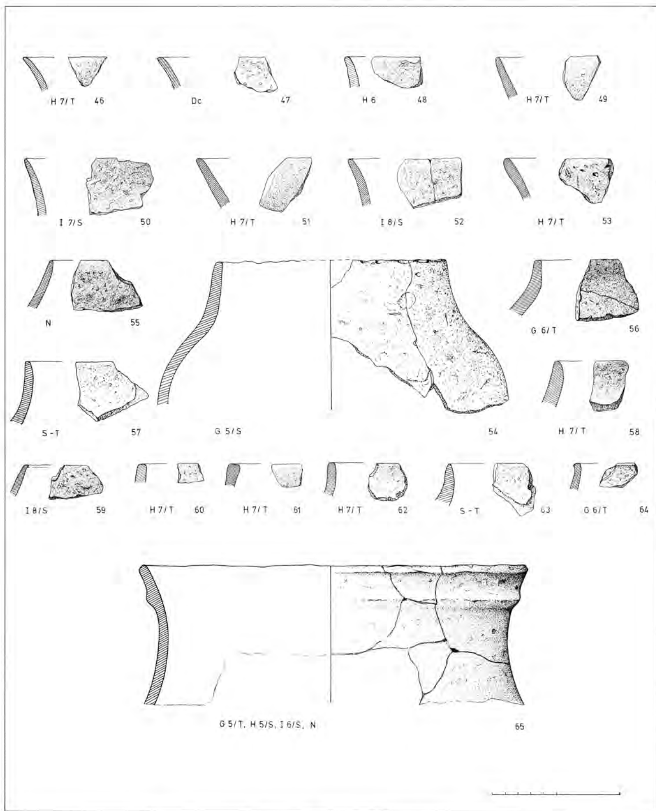
FIG. 48. — Céramique néolithique : gobelets (46-64); jarre à provisions (65)
