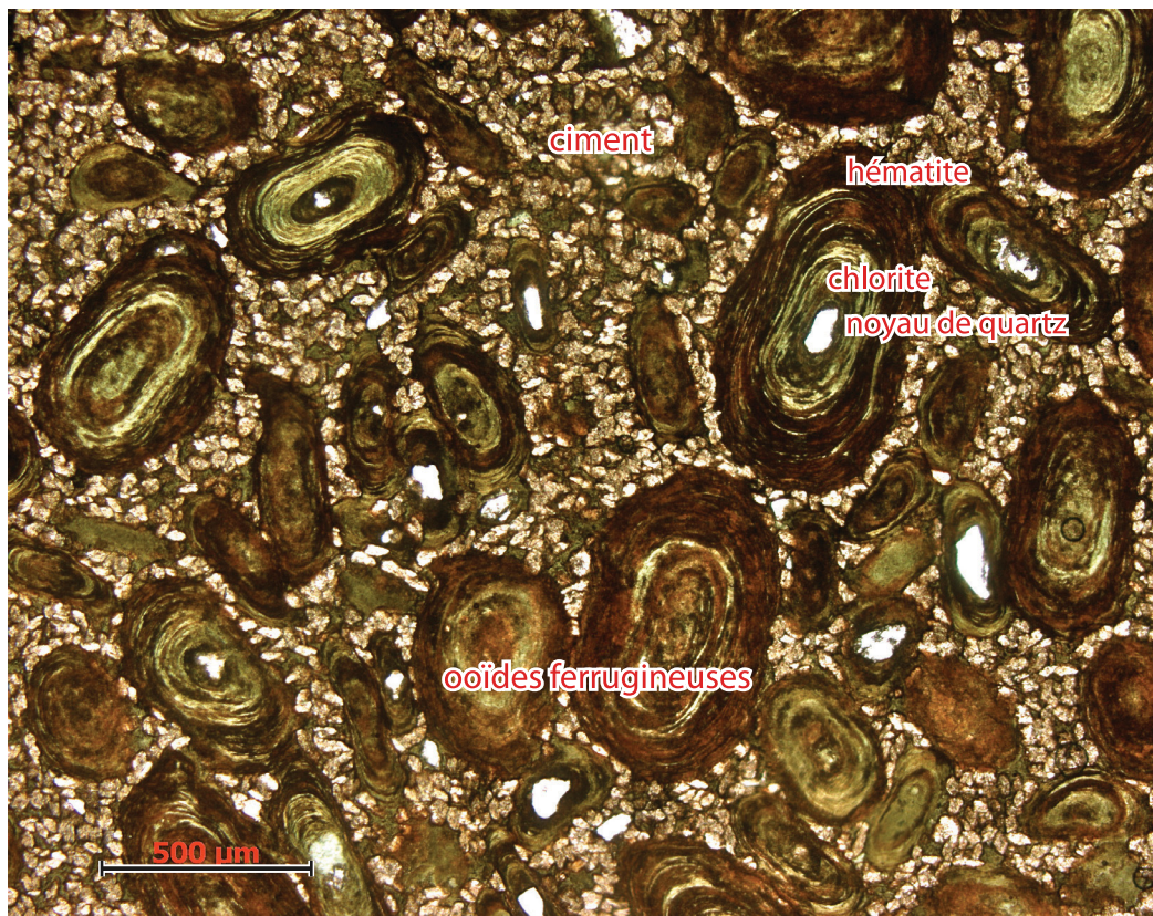
Fig. 4 – Photographie au microscope polarisant du minerai oolithique montrant des oïdes ferrugineuses à alternance de lamines hématitique (brun rouge) et chloritique (vert). Le ciment est composé de chlorite et de rhomboédres de sidérite.
