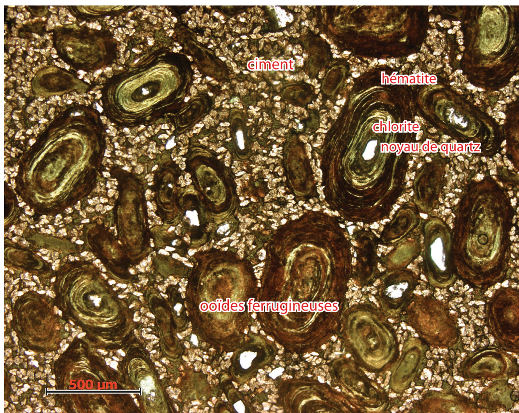
Fig. 4 – Photographie au microscope polarisant du minerai oolithique montrant des oôïdes ferrugineux à alternance de lamines hématitiques (brun rouge) et chloritiques (vert). Le ciment est composé de chlorite et de rhomboédres de sidérite.
