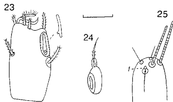
FIG. 23-25. — Ereynetes exilis Fain et Prasse, femelle : tarse I (23); E. malayi Fain et al., femelle : tarse palpal (24); Dermatophagoides farinae Hughes, femelle : extrémité apicale du tarse I dorsalement (25). (Remarque : L' échelle mesure 0,01 mm)
