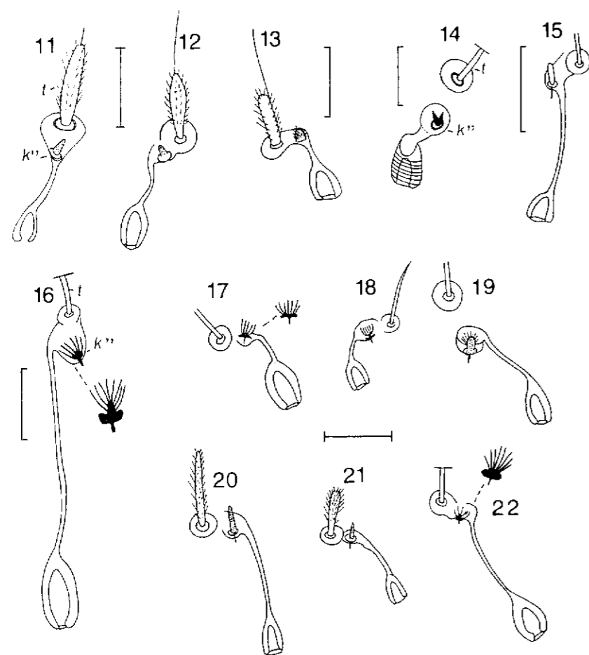
FIG. 11-22. — Organe ereynetale du type A chez divers Speleognathinae : Spelcorodens derricki (Womersley), femelle (11) ; Paraspeleognathopsis bakeri (FAIN), femelle (12) ; P. galagoensis (Fain), femelle (13) ; Speleognathus australis Womersley, femelle (14) ; Speleomyotis bastini (Fain), femelle (15) ; Neoboydaia philomachi (Fain), femelle (16) ; Metaboydaia poffei (Fain), femelle (17) et larve (18) ; Phoenicopteriella womersleyi (Fain), femelle (19) ; Boydaia indica Fain, femelle (20) et larve (21) ; Speleognathopsis benoiti Fain, femelle (22).
