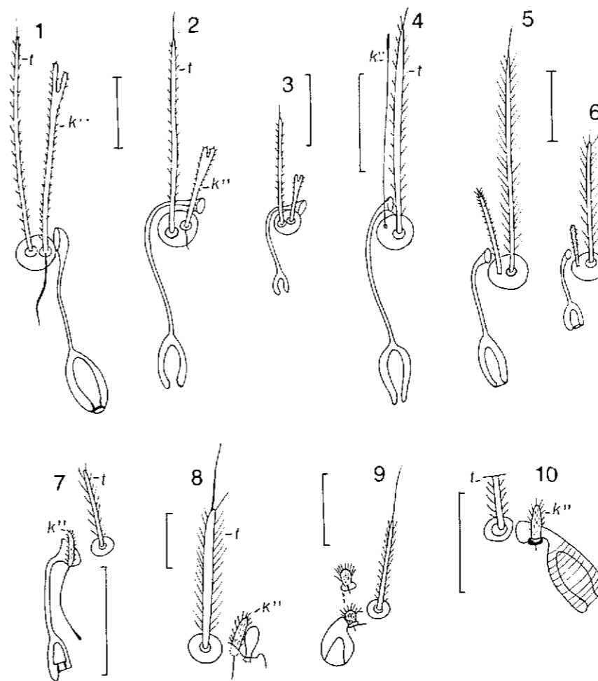
FIG. 1-10. : FIG. 1-6. — Organe ereynetal du type B chez divers Ereynetinae : Riccardoella oudemansi Sig Thor, femelle (ex Arion rufus ) (1) ; R. limacum (Schrank), femelle (ex Helix aspersa ) (2) et larve (ex Helicella sp.) (3) ; Ereynetes hydrophilus Cooreman, femelle (4) ; E. papuanus Fain et al., femelle (5) et larve (6).
