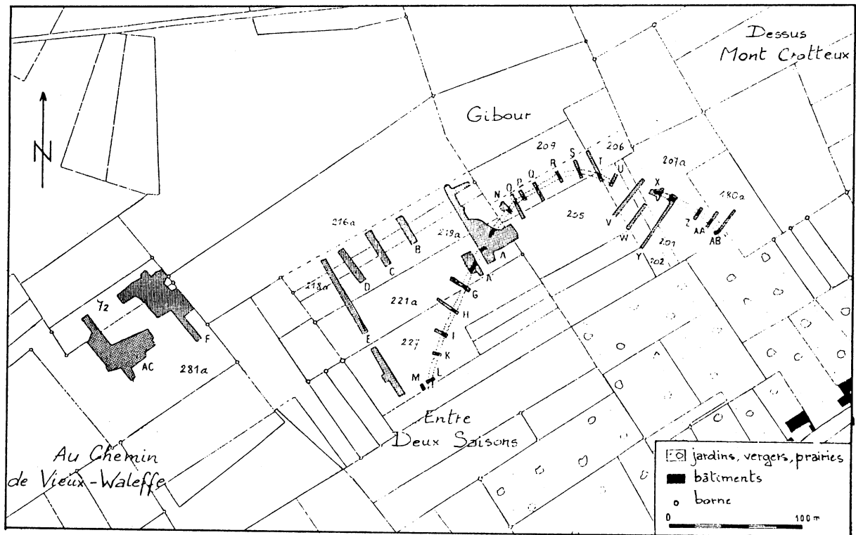
Fig. 1 - 1 : situation topographique du site de Vaux-et-Borset «Gibour»; 2 : plan général des fouilles. Les tranchées sont figurées en grisé.
