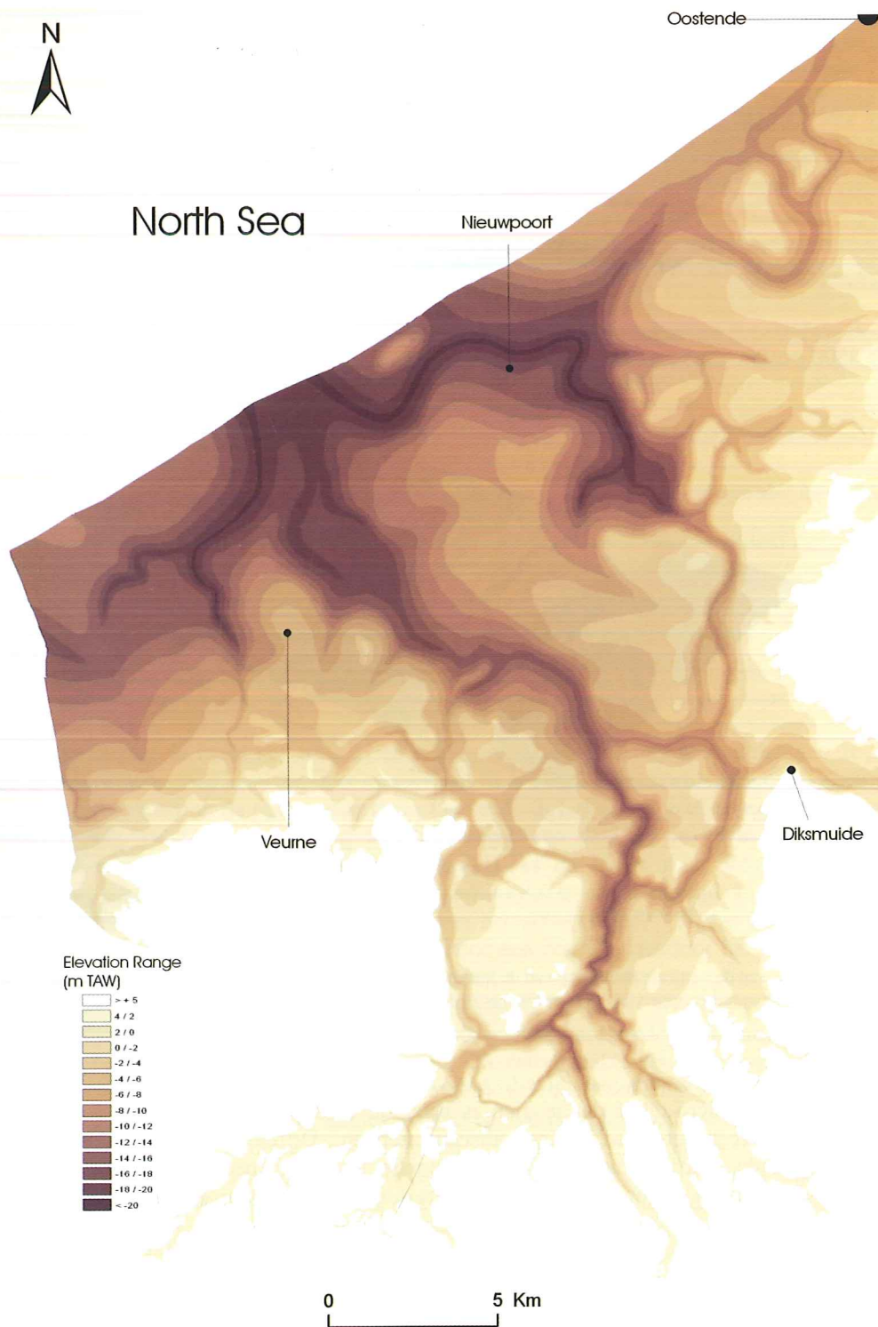
Fig. 3.8 Reliëfkaart van de basis van de Holocene sedimenten waarop de verticale insnijding van de jonge getijgeulen tot uiting komt (vergelijk met Fig. 3.1).
