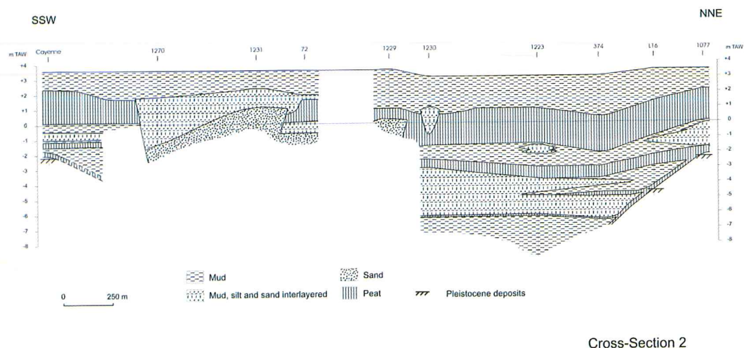
Fig. 5.4 Dwarsdoorsnede 2.
