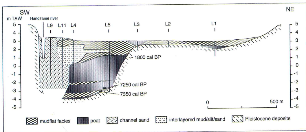
Fig. 5.5 Dwarsdoorsnede van de paleovallei van de Handzame.
