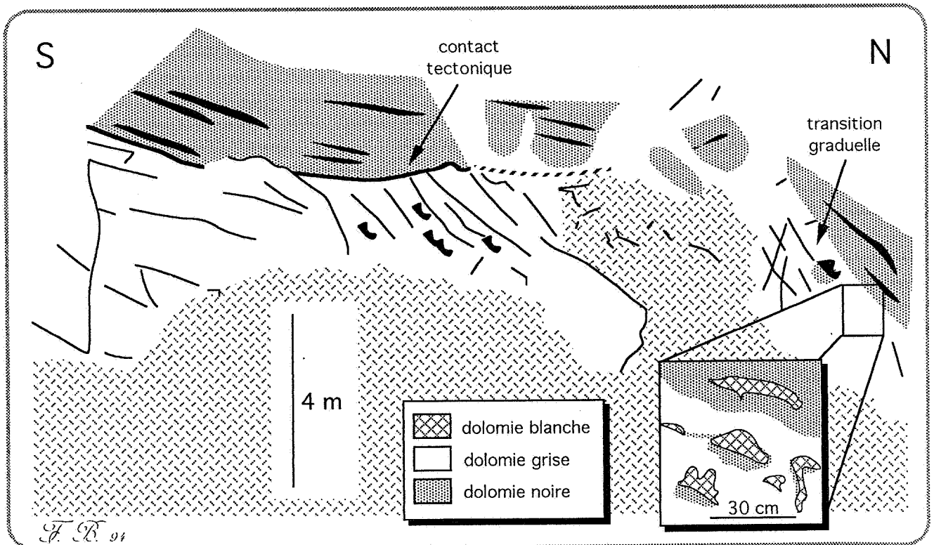
fig. 7: contact anormal entre des dolomies grises à fenestrac et des dolomies noires zébrées. Base de la coupe du front 3
