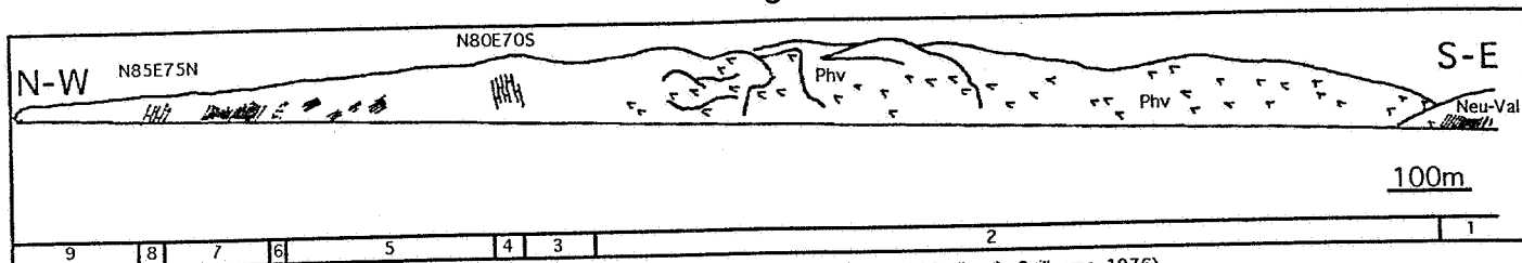
Coupe G4: le long de la route de Villers-Le-Gambon à Givet, à hauteur du Bois de Rinval (affl.16900-09600-pl.10, d'après Guillaume, 1976)
