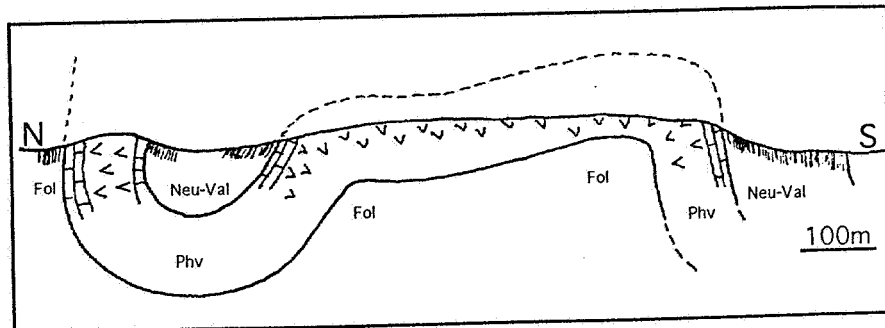
Fig.3: coupes géologiques tirées des travaux de Thonnard (1964) et Guillaume (1976)
