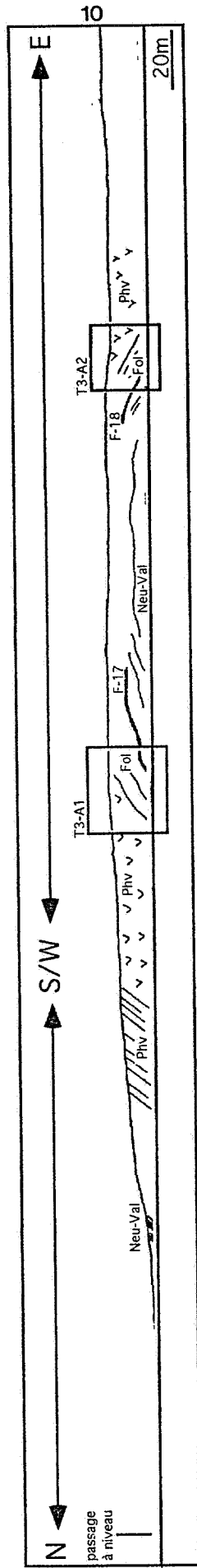
Coupe T3A: le long de l'ancien chemin de fer de Merlemont (affi.104-pl.46, d'après Thonnard, 1964).
