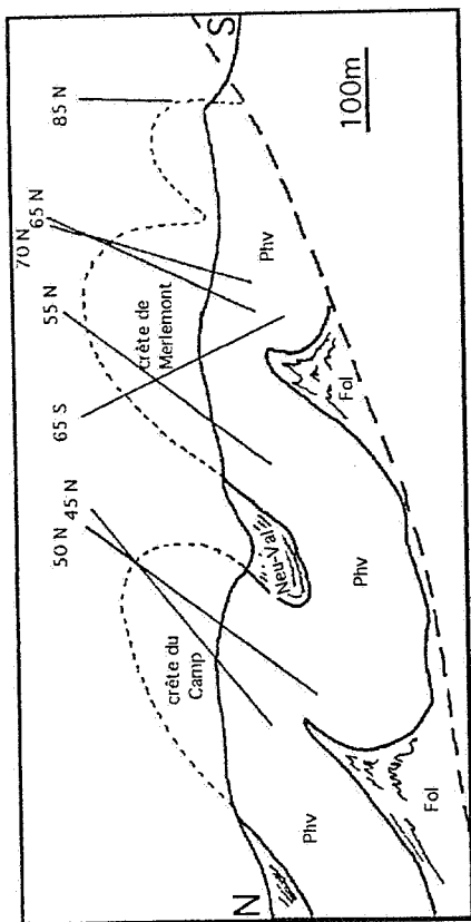
Coupe T2B: interprétation donnée par Thonnard (1964) des observations effectuées à la coupe T2A
