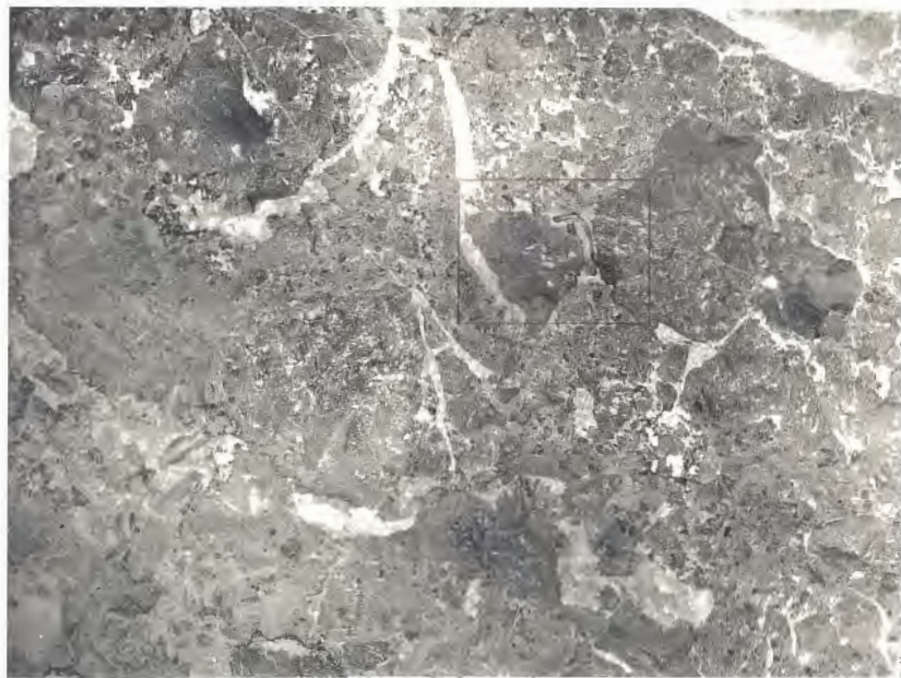
FIG. 1. — Aphrostroma tenerum , Gürich, 1906. — Viséen (V 2 d).
