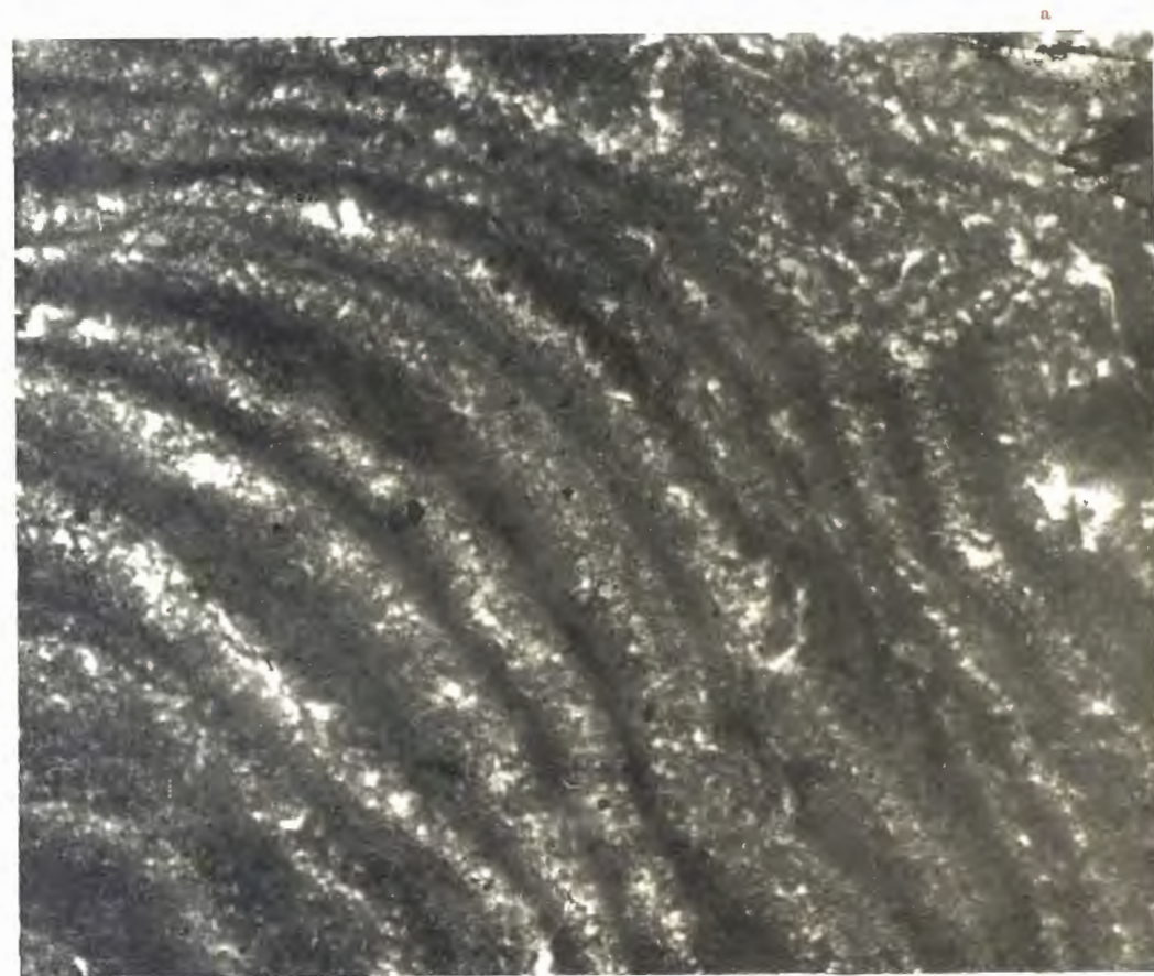
FIG. 2. — Malacostroma concentricum , Gürich, 1906. — Viséen (V 2 b).
