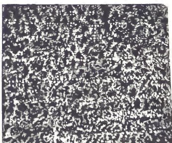
FIG. 2 Pycnostroma densius , Gürich, 1906. Grands-Malades. Petite plaque mince. — Cliché 47. Grossissement : 50 (environ).
