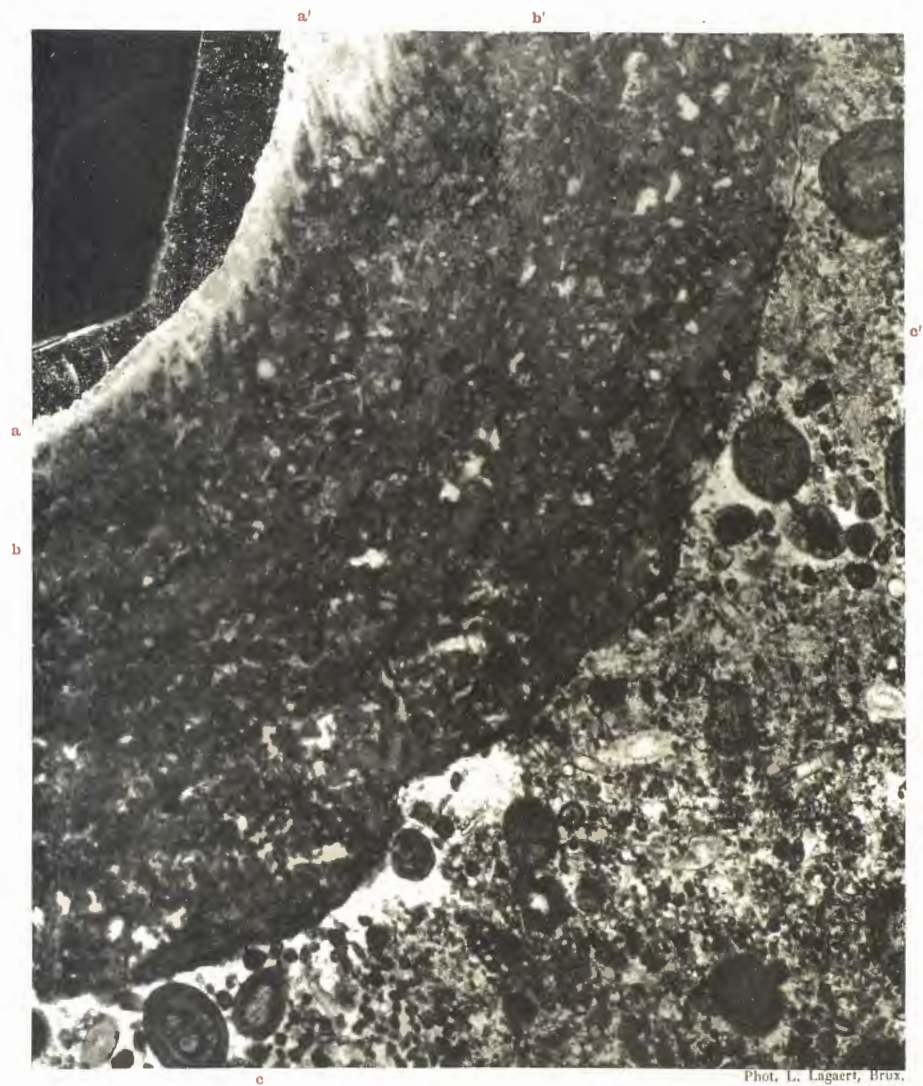
FIG. 2. — Pycnostroma spongilliferum , Gürich, 1906. — Viséen (V 2 d). Andenne. — Plaque mince 52. — Grossissement : 20. — Calcaire carbonifère. Type : Musée de Bruxelles.
