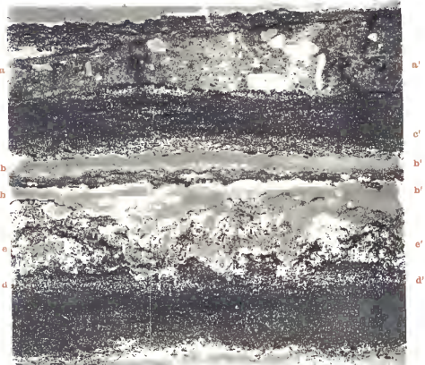
FIG. 1. — Spongiostroma bacilliferum , Gürich, 1906. — Viséen (V 2 d). Namèche. — Plaque 249. — Grossissement : \frac{1}{2} . — Calcaire carbonifère. Type : Musée de Bruxelles.
