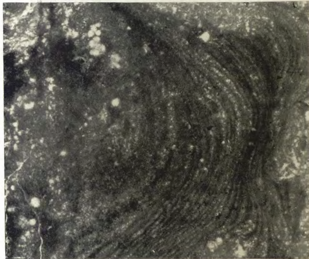
FIG. 2. — Malacostroma concentricum , Gürich, 1906. — Viséen (V 2 b).
