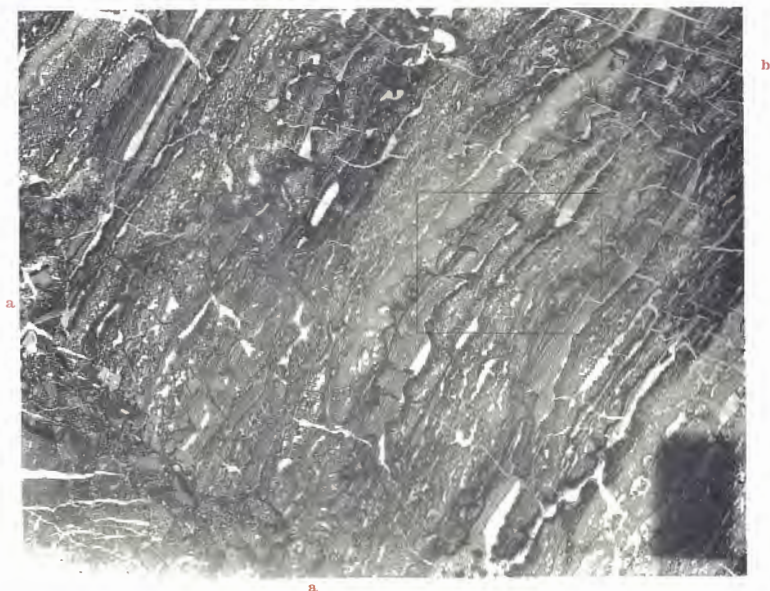
FIG. 1. — Chondrostroma globuliferum , Gürich, 1906. — Viséen (V 2 b). Grands-Malades. — Plaque 253. — Grandeur naturelle. — La région encadrée de rouge est celle grossie dans la figure 2. Type : Musée de Bruxelles.
