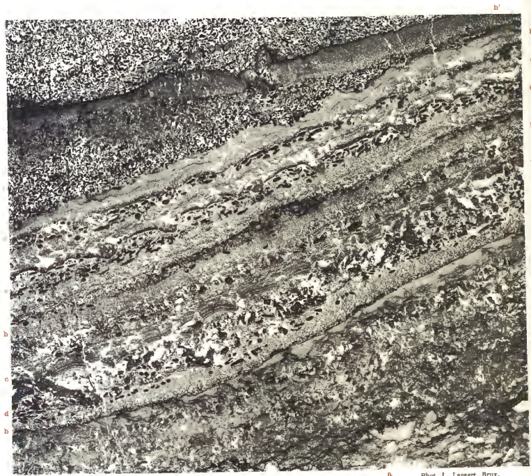
FIG. 3. — Spongiostroma ovuliferum , Gürich, 1906. — Viséen (V 2 b). F. Champion (6998). — Plaque 9 x 13 cm. — Grossissement : 5. — Calcaire carbonifère. Type : Musée de Bruxelles.
