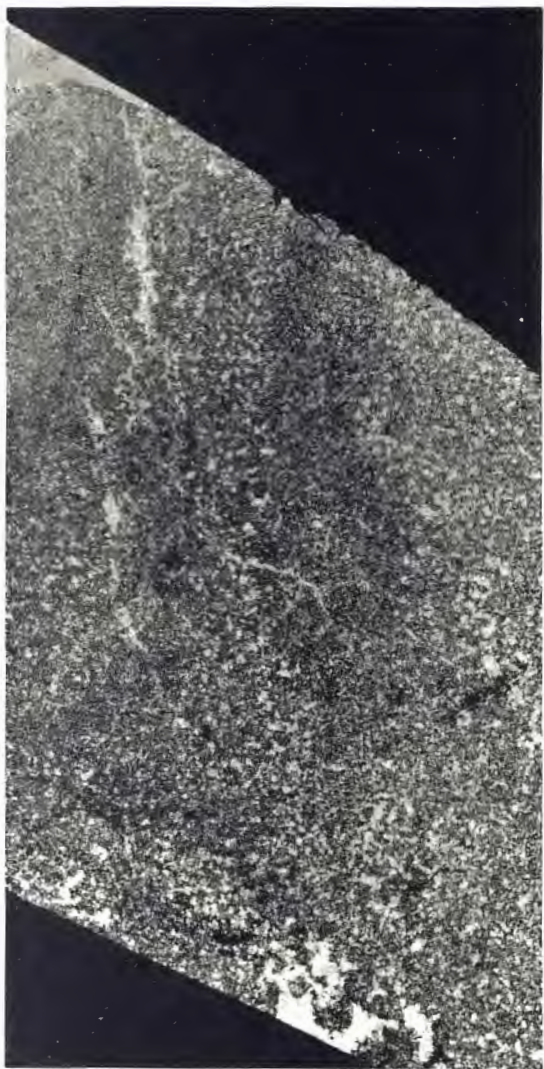
FIG. 1. — Malacostroma concentricum , Gürich, 1906. — Viséen (V 2 b).
