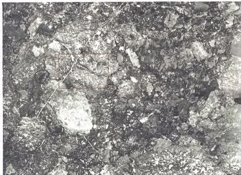
FIG. 1. — Aphrostroma tenerum , Gürich, 1906. — Viséen (V 2 c).
