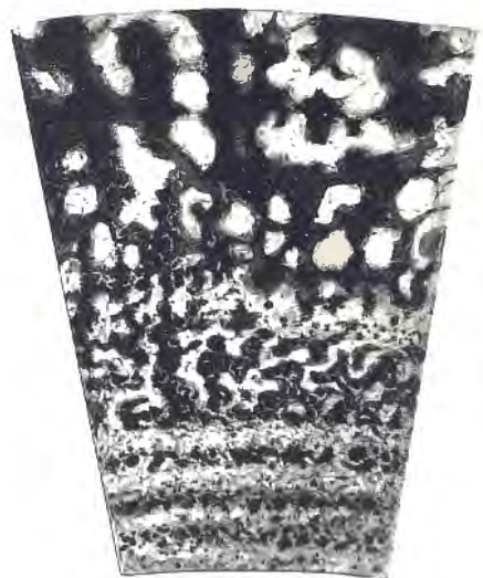
FIG. 1. Aphrostroma tenerum , Gürich, 1906. Namèche. Plaque 217. — Cliché 81. Grossissement : 50 (environ).
