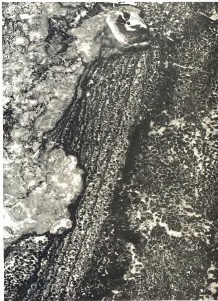
FIG. 3. — Chondrostroma problematicum , Gürich, 1906. — Viséen (V 2 b). Modave à Barse. — Plaque 303. — Grossissement : 20. — Calcaire carbonifère.
