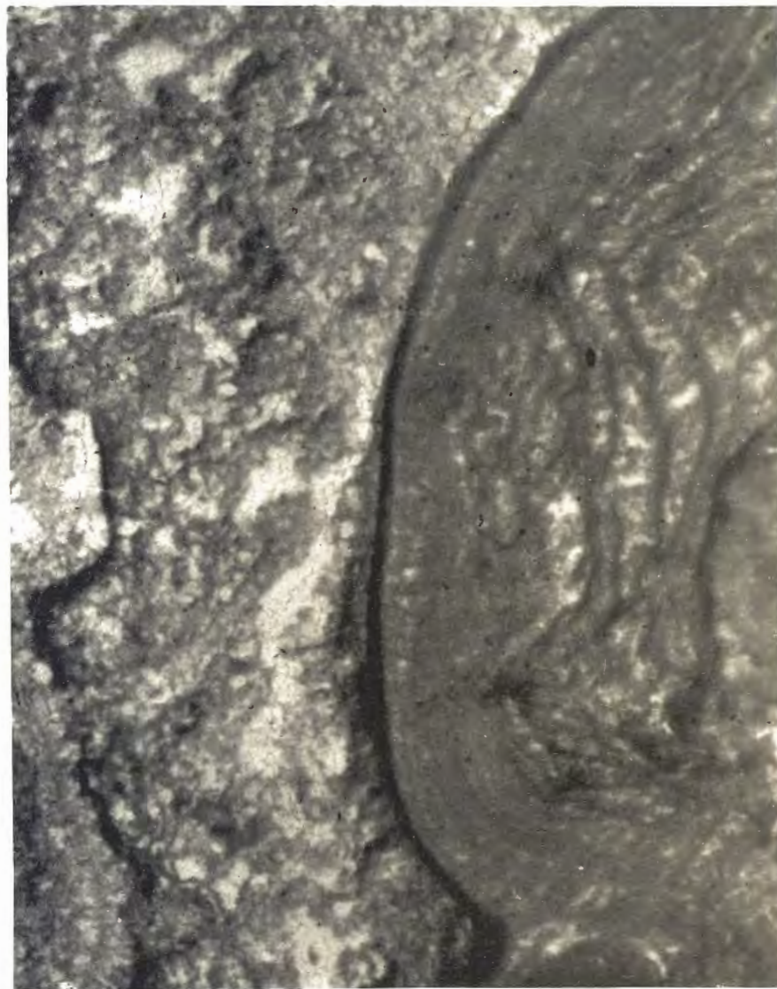
FIG. 2. — Malacostroma undulosum , Gürich, 1906. — Viséen (V 2 b).
