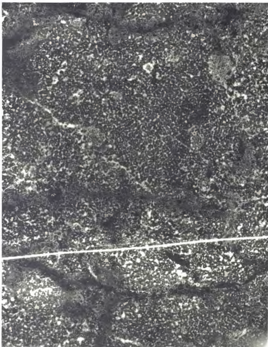
FIG. 1. — Spongiostroma mæandrinum , Gürich, 1906. — Viséen (V 2 d). Namèche. — Plaque 229. — Grossissement : 20. — Calcaire carbonifère. Type : Musée de Bruxelles.
