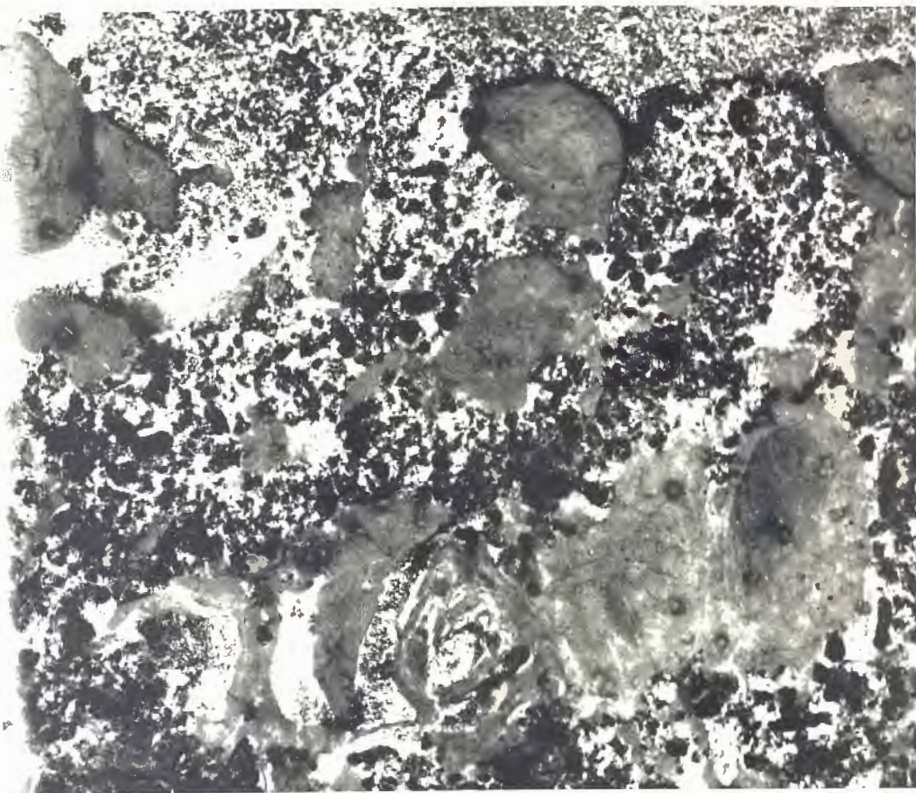
FIG. 1. — Nodules stéréoplasmiques. — Viséen (V 2 d). Namèche. — Plaque 240. — Grossissement : 20. — Calcaire carbonifère. Collections du Musée de Bruxelles.
