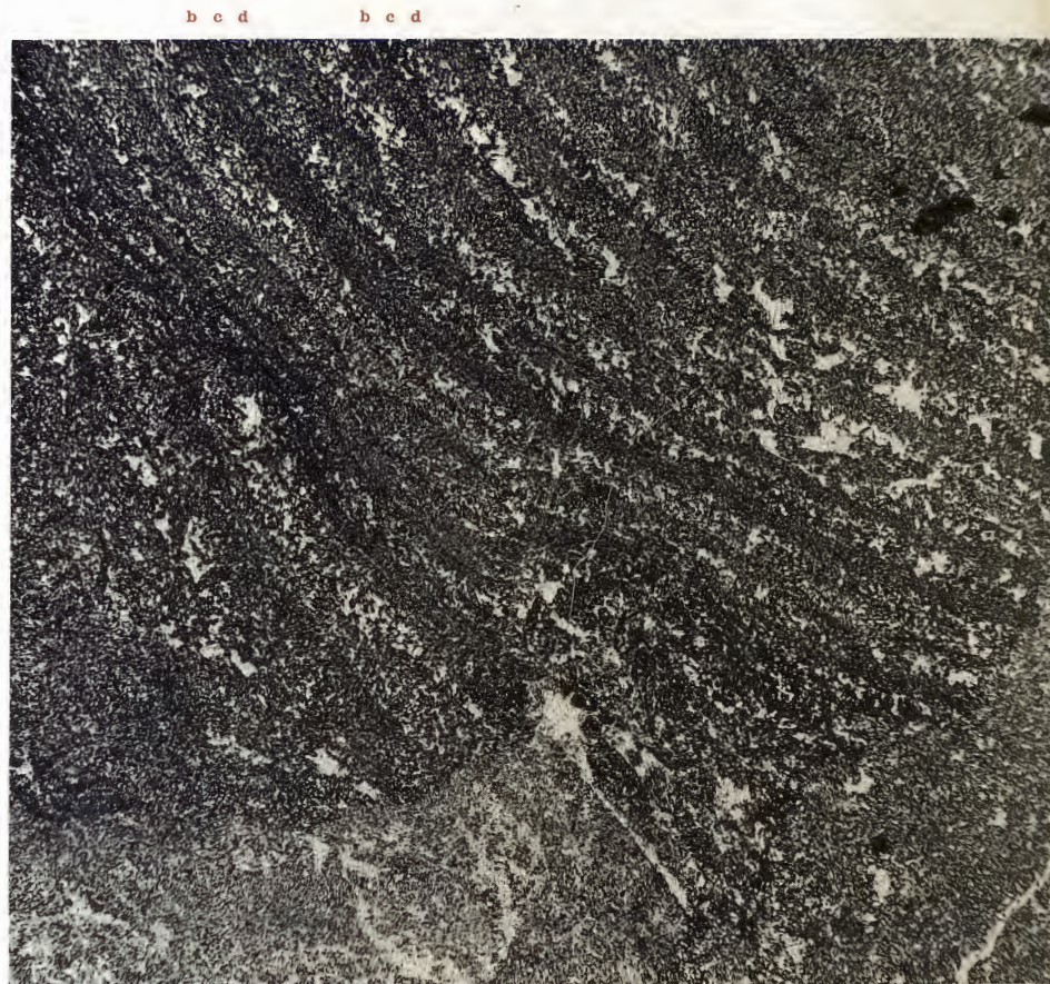
FIG. 2. — Malacostroma concentricum , Gürich, 1906. — Viséen (V 2 b).
