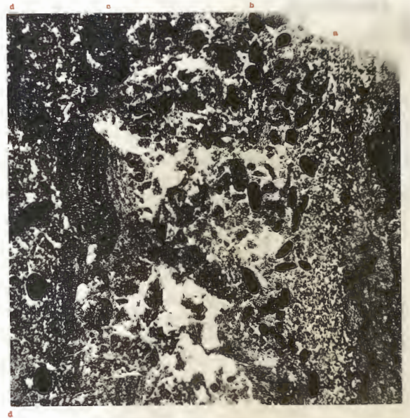
FIG. 2. — Spongiostroma ovuliferum , Gürich, 1906. — Viséen (V 2 d). Namèche. — Même plaque. — Grossissement : 20. — Coupe verticale. Type : Musée de Bruxelles.
