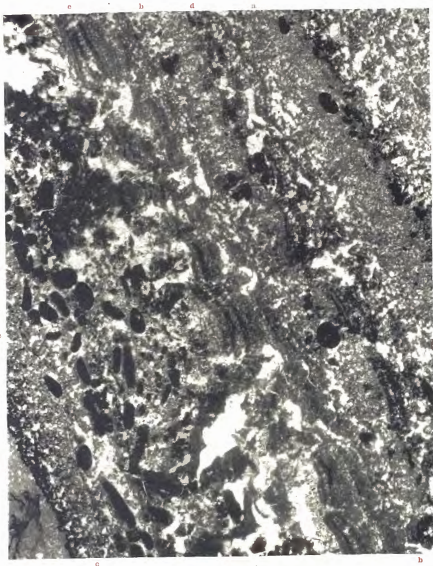
FIG. 1. — Spongiostroma ovuliferum , Gürich, 1906. — Viséen (V 2 d). Namèche. — Plaque 9 × 12 cm. — Grossissement : 20. — Coupe verticale. Type : Musée de Bruxelles.
