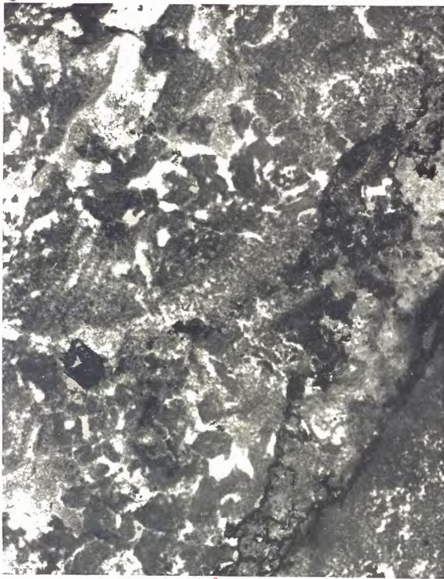
FIG. 1. — Calcaire à Stylolithes. — Viséen (V 2 c).
