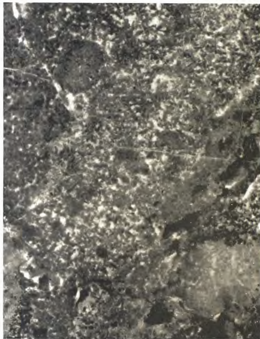
FIG. 3. — Chondrostroma intermixtum , Gürich, 1906. — Viséen (V 2 b). Grands-Malades. — Plaque 253. — Grossissement : 20. — Calcaire carbonifère. Type : Musée de Bruxelles.
