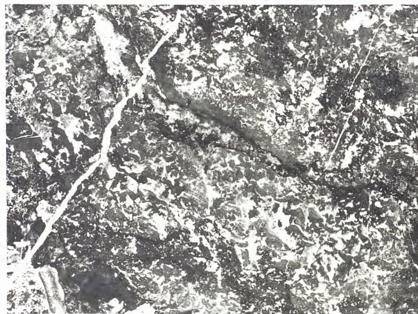
FIG. 2. — Aphrostroma tenerum , Gürich, 1906. — Viséen (V 2 c).
