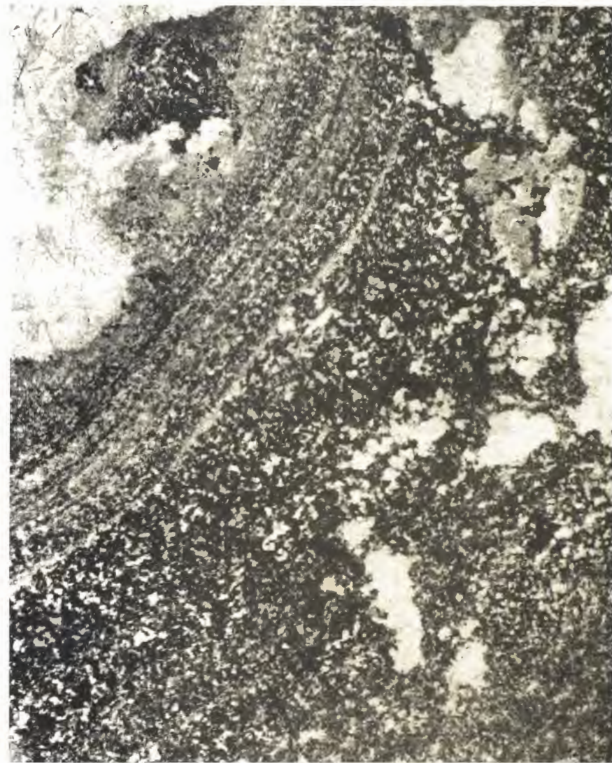
FIG. 3. — Aphrostroma tenerum , Gürich, 1906. — Viséen (V 2 d).
