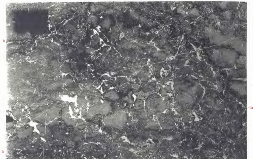
FIG. 1. — Chondrostroma vermiculiferum , Gürich, 1906. — (Viséen V 2 b). Herbatte. — Plaque 242. — Grandeur naturelle. — Calcaire carbonifère. Type : Musée de Bruxelles.
