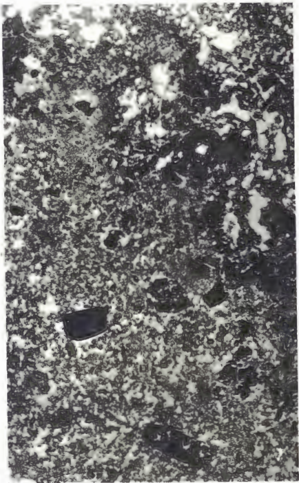
FIG. 1. — Spongiostroma ovuliferum , Gürich, 1906. — Viséen (V 2 d). Namèche. — Plaque 9 x 13 cm. — Grossissement : 20. — Coupe horizontale. Type : Musée de Bruxelles.
