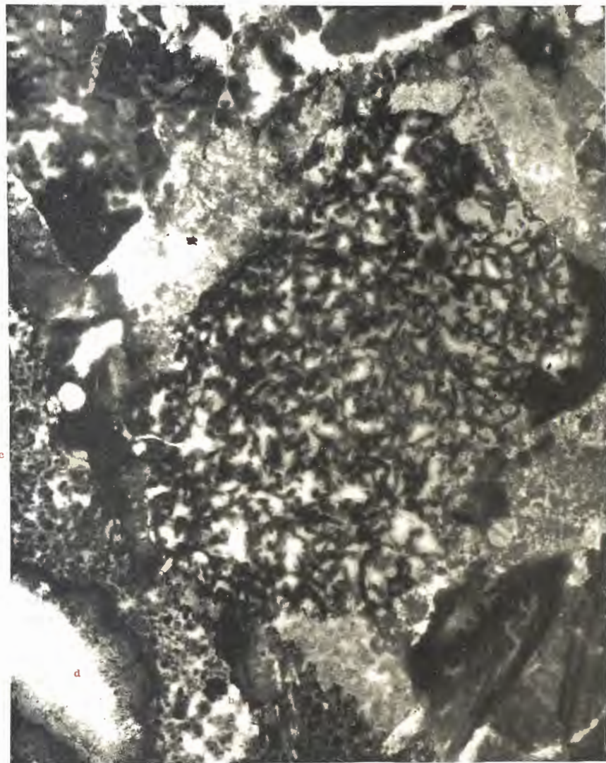
FIG. 3. — Chondrostroma vermiculiferum , Gürich, 1906. — Viséen (V 2 b). Herbatte. — Plaque 241. — Grossissement : 20. — Calcaire carbonifère. Type : Musée de Bruxelles.
