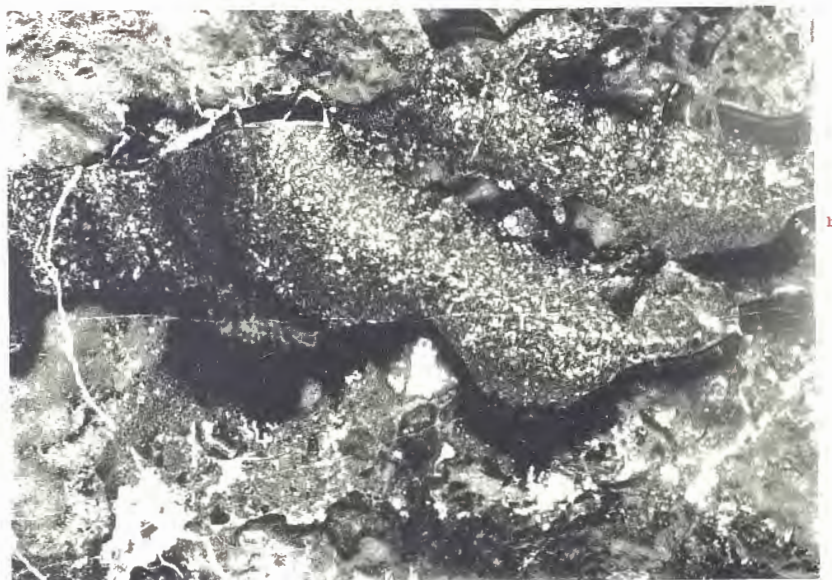
FIG. 2. — Chondrostroma vermiculiferum , Gürich, 1906. — Viséen (V 2 b). Herbatte. — Plaque 242. — Grossissement : 5. — Calcaire carbonifère. Type : Musée de Bruxelles.
