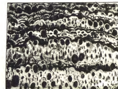
FIG. 5. Chondrostroma problematicum , Gürich, 1906. Modave à Barse. Plaque 303. — Cliché 63 (coupe verticale). Grossissement : 50 (environ).
