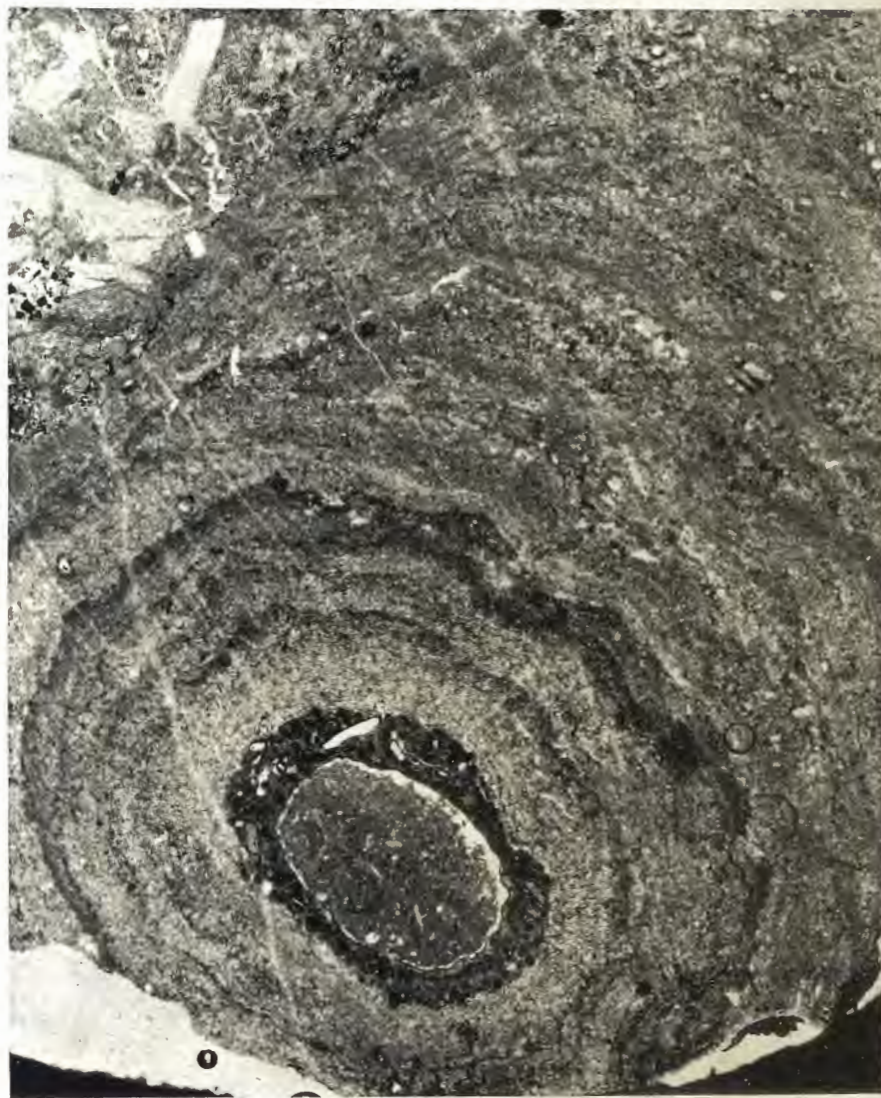
FIG. 2. — Pycnostroma densius , Gürich, 1906. — Viséen (V 2 b). Grands-Malades. — Plaque mince 48. — Grossissement : 20. — Calcaire carbonifère. Type : Musée de Bruxelles.
