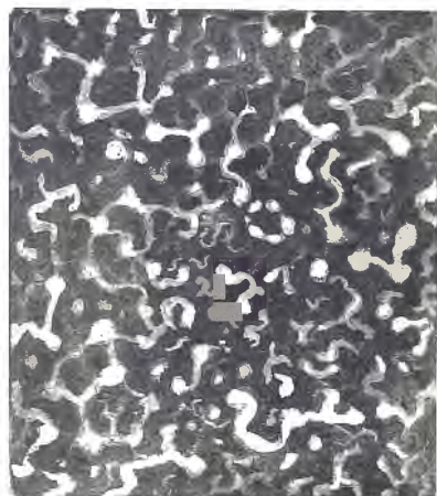
FIG. 3. Spongiostroma mæandrinum , Gürich, 1906. Namèche. Plaque 229. — Cliché 64 (coupe horizontale). Grossissement : 50 (environ).
