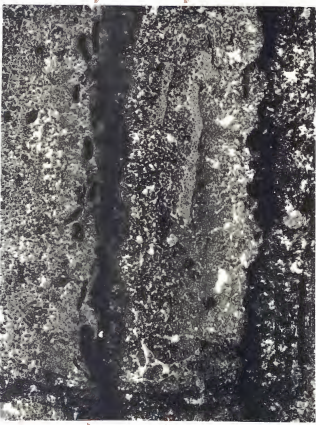
FIG. 1. — Spongiostroma bacilliferum , Gürich, 1906. — Viséen (V 2 d). Namèche. — Plaque 240. — Grossissement : 20. — Calcaire carbonifère. Type : Musée de Bruxelles.
