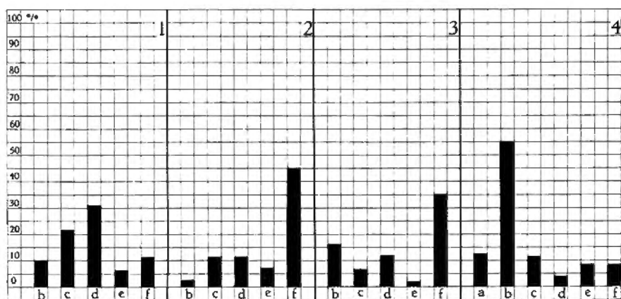
Fig. 2. — Granulométrie du sol : a = > 1 mm. b = 0,2 - 1 mm. c = 0,1 - 0,2 mm. d = 0,05 - 0,1 mm. e = 0,02 - 0,05 mm. f = < 0,02 mm.
