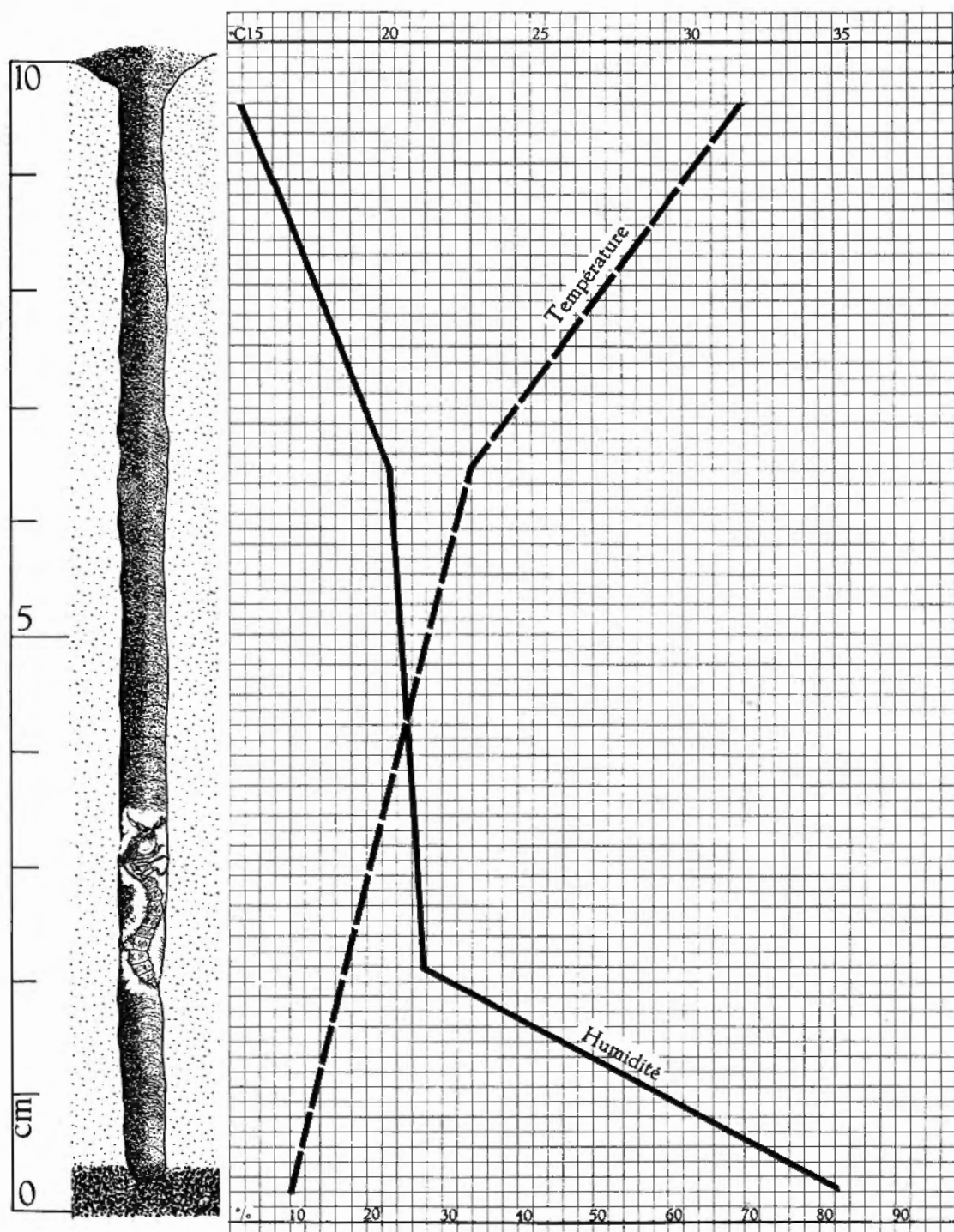
Fig. 15. — Profil de la galerie de la larve de Cicindela hybrida L.
