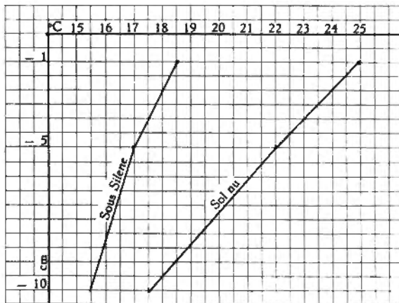
Fig. 6. — Profils thermiques sous une plante et dans le sol découvert.
