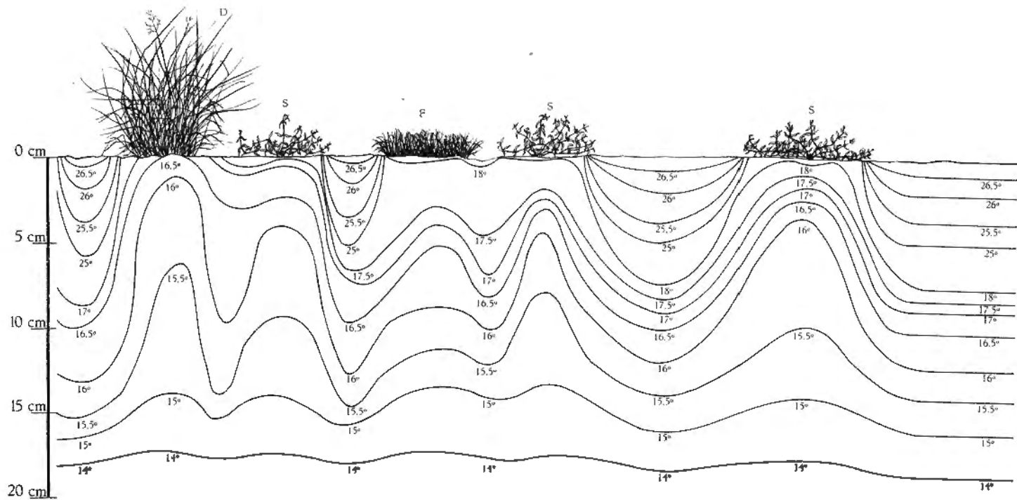
Fig. 4. — Profil thermique du sol dans le groupement végétal colonisateur.
