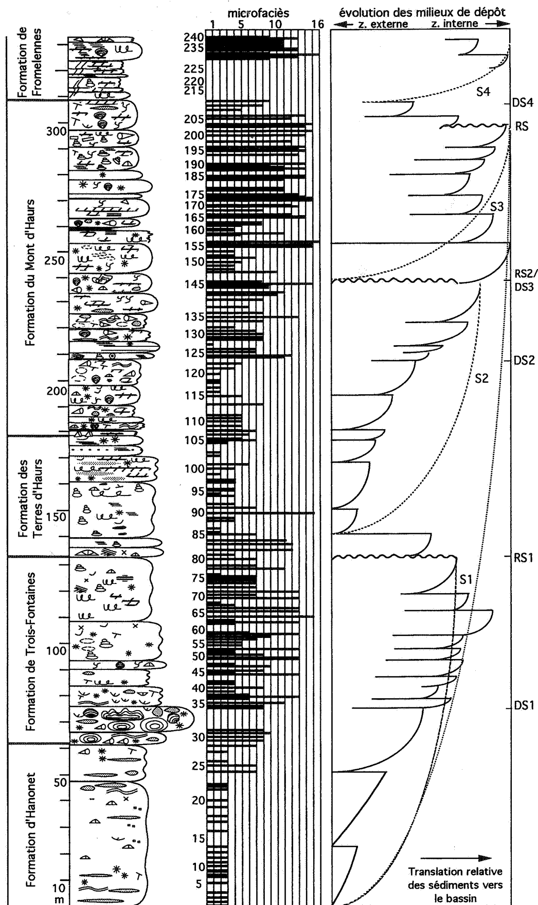
Figure 9. Colonne lithologique, microfaciès et interprétation séquentielle du Givetien de Glageon. S1-4: séquences pluridécamétriques; RS: surface de ravinement; DS: surface marquant le maximum de vitesse de translation des sédiments vers le bassin (downward shift).
