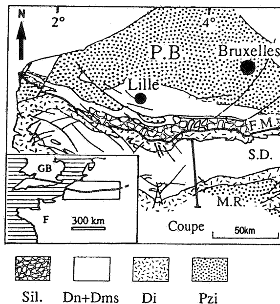
Figure 2a. Situation régionale. P.B.: Parautochtone brabançon; F.M.: Faille du Midi; S.D.: Synclinorium de Dinant; M.R.: Massif de Rocroi. Sil.: Silésien; Dn+Dms: Dinantien et Dévonien moyen et supérieur; Di: Dévonien inférieur; Pzi: Paléozoïque inférieur.
