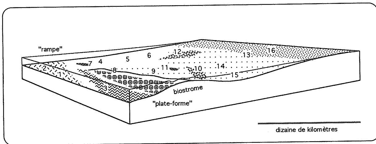
Figure 8. Répartition des microfaciès (1-16) du Givetien de Glageon par rapport à un modèle simple de plate-forme asymétrique.
