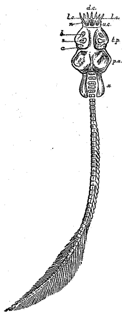
FIG. 5. — Palaeospondylus .
