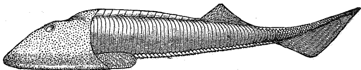
Fig. 12. — Cephalaspis Murchisoni . RESTAURATION DEMI-GRANDEUR.
