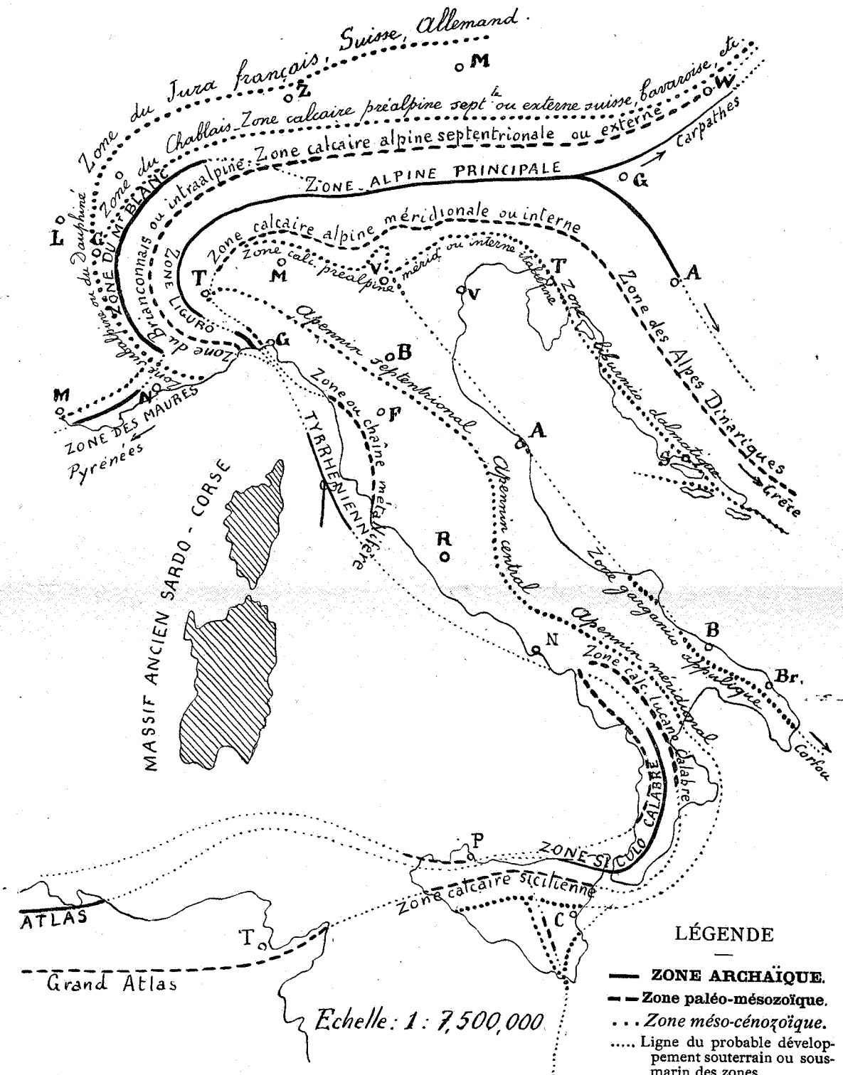
F. SACCO. — SCHÉMA GÉOTECTONIQUE DES ALPES ET DE L'APENNIN.
