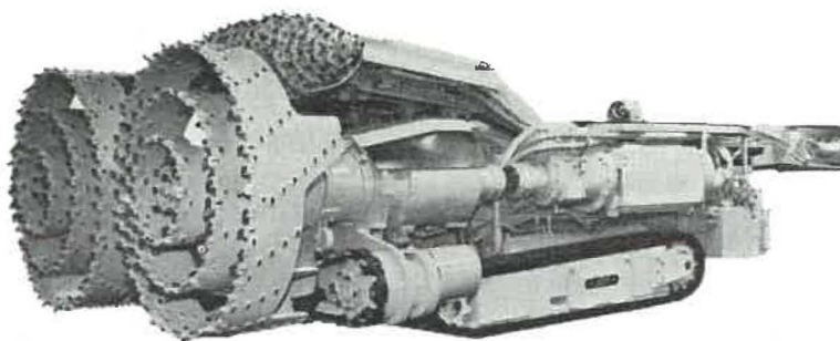
Fig. 7. — Mineur continu circulaire Joy CU-61 Compton.
