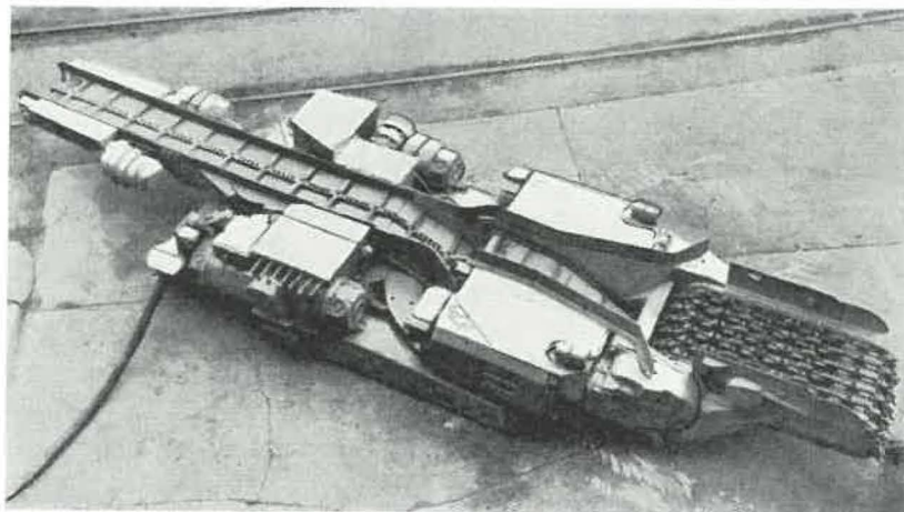
Fig. 12. — Plan d'ensemble du convoyeur Joy extensible.
