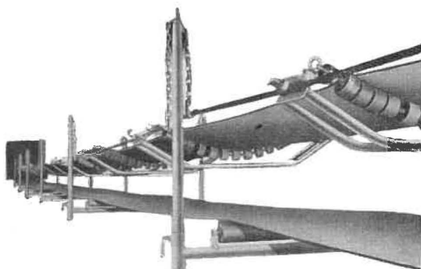
Fig. 15. — Le convoyeur Limberope à support par câble acier.
