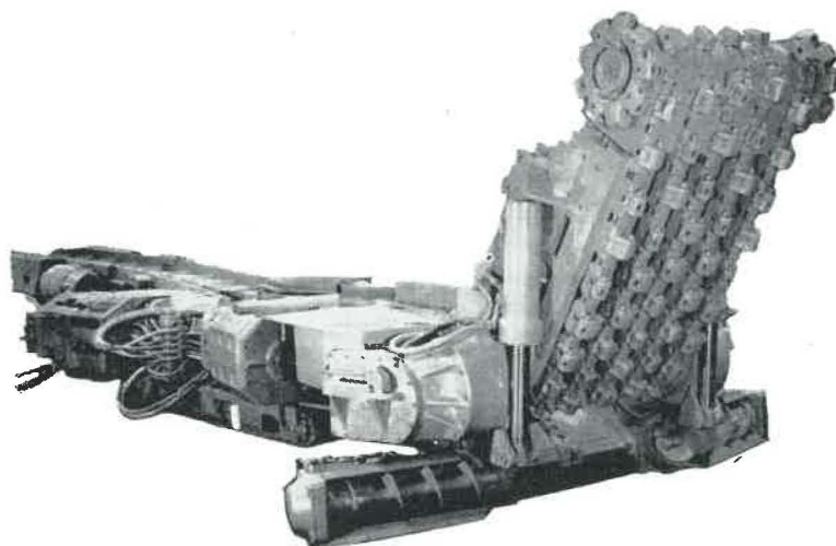
Fig. 1. — Mineur continu Joy 5-CM pour couches minces ou moyennes.
