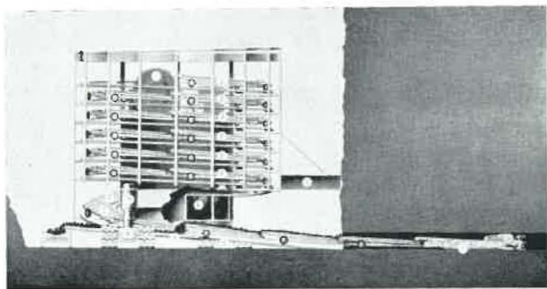
Fig. 9. — Schéma du principe de fonctionnement du mineur Joy télécommandé vu de profil.
