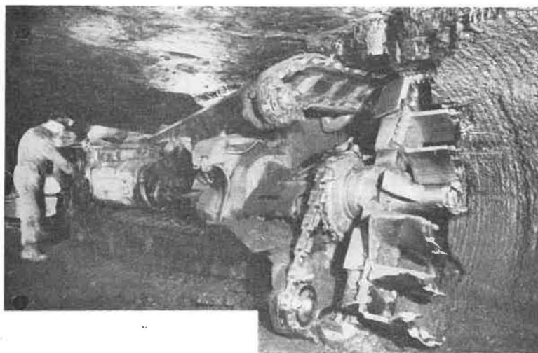
Fig. 6. — Mineur continu Joy à deux têtes rotatives type 2-BT-2.
