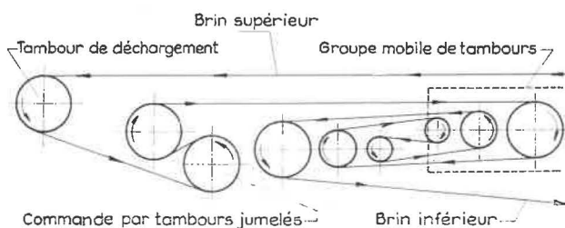
Fig. 13. — Schéma du dispositif d'emmagasinement de bande.
