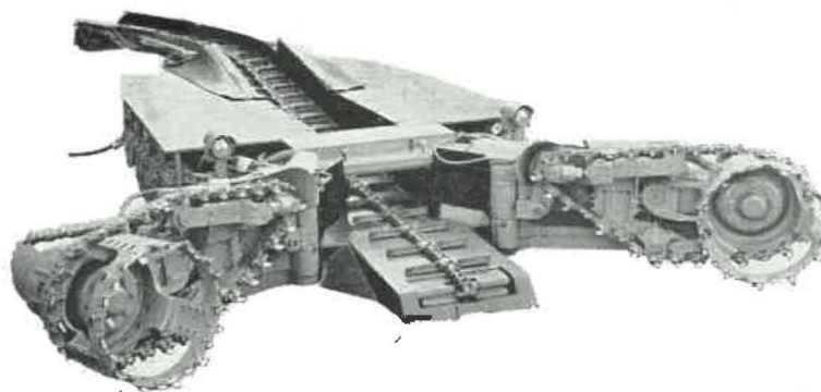
Fig. 3. — Le mineur continu Joy CU-42 Compton pour couches minces n'a qu'une hauteur de 760 mm. Ses têtes de havage circulaires montées sur bras articulés produisent une forte proportion de gaillettes.
