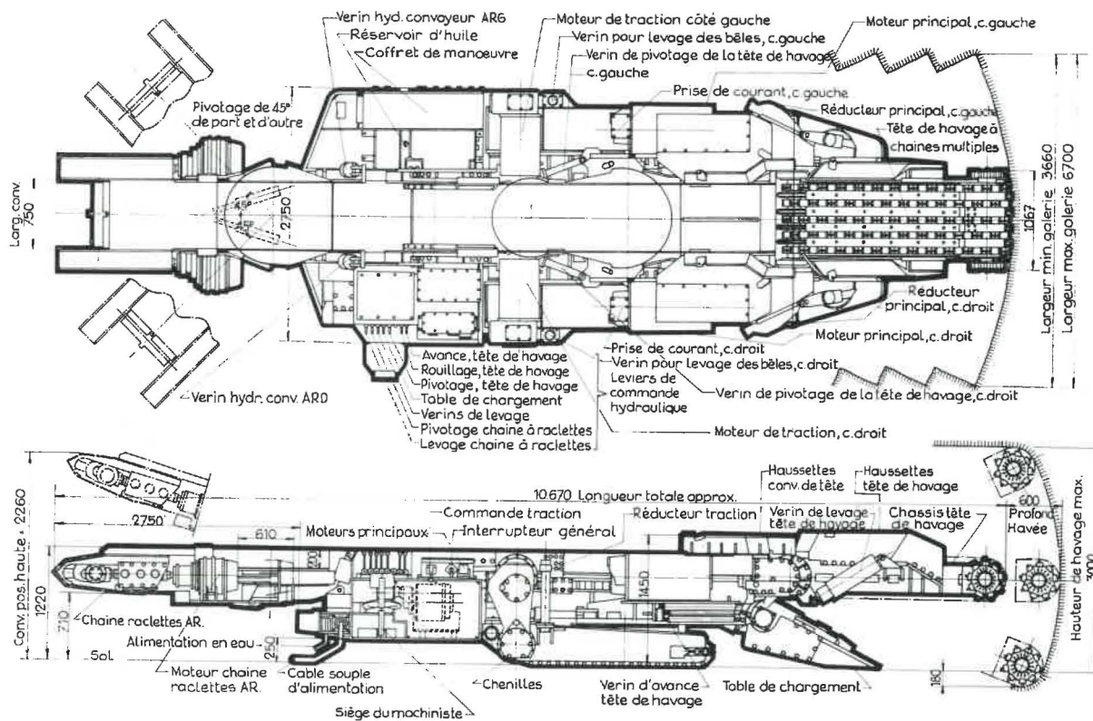
Fig. 2. — Plan d'ensemble du mineur continu Joy 6-CM.
