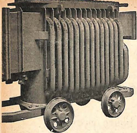
Transformateur anti-déflagrant pour mine grisouteuse — Type TID. 27 R.
