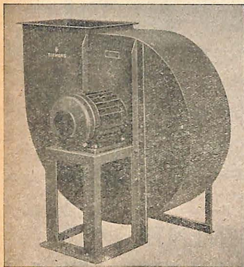
VENTILATEUR CENTRIFUGE
