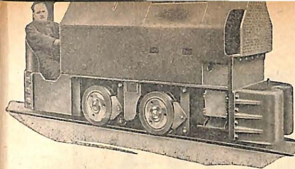
Modèle DLM.2 de 28 CV.
